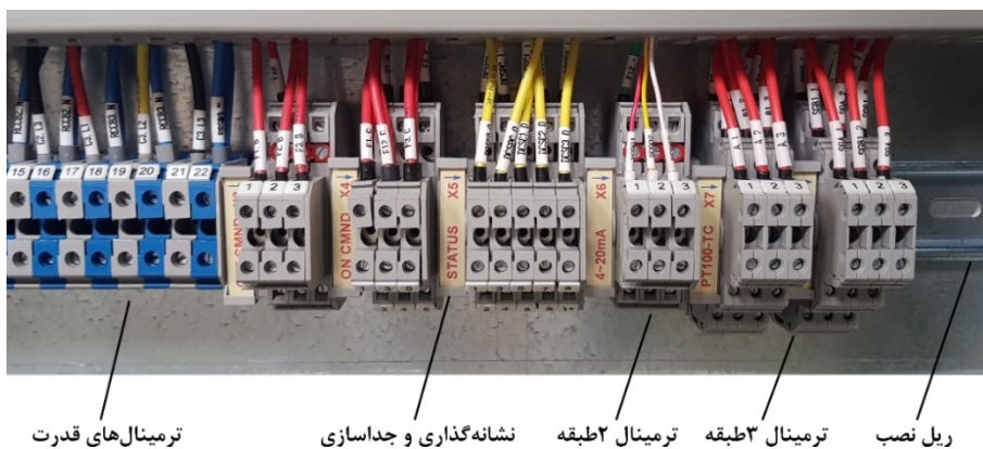
شکل ۶-۵۱- بلوک ترمینال با جداسازی و علامتگذاری بخش‌های مختلف
