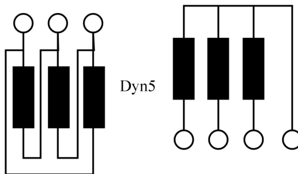
شکل ۸-۱- الف) گروه برداری Dyn5
