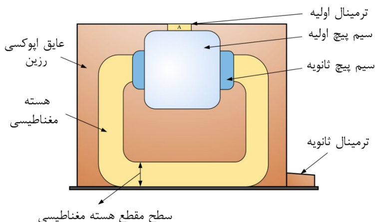
شکل ۷-۱۰- نمای شماتیک ترانسفورماتور ولتاژ تک‌فاز (که بین یک‌فاز و زمین قرار می‌گیرد)
