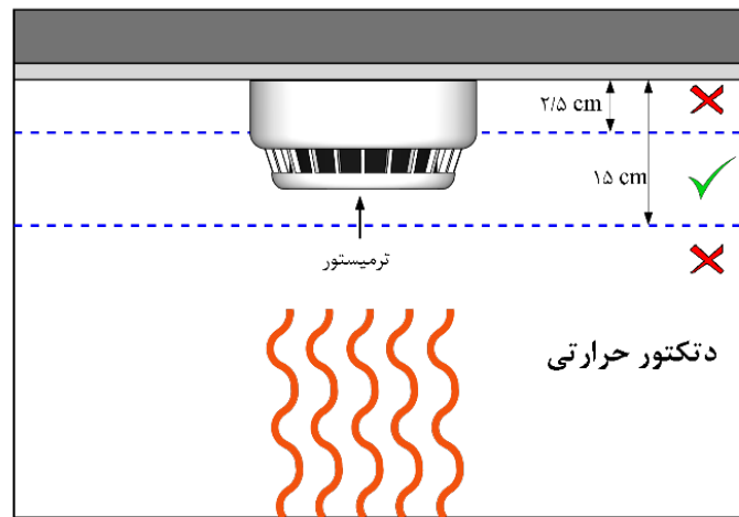
شکل ۴-۳۷- محدود مجاز جانمایی دکتور حرارتی
