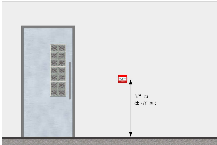
شکل ۴-۲۸- حدود ارتفاع مجاز جانمایی شستی اعلام حریق
