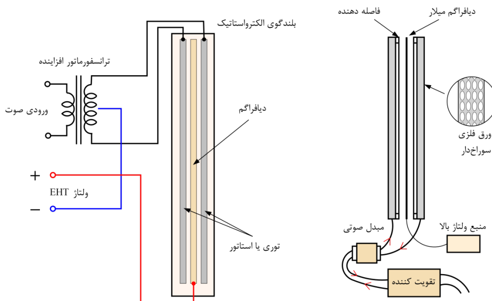
شکل ۷-۱۱۰- ساختمان داخلی یک واحد راه‌انداز بلندگوی الکترواستاتیک
