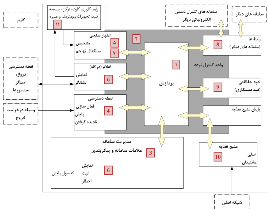
شکل ۳-۳۳- معماری عمومی سیستم کنترل دسترسی الکترونیکی
