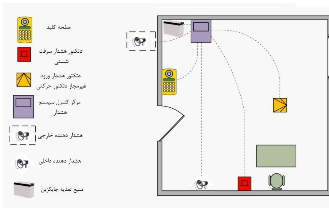
شکل ۳-۳- شمایی ساده از جانمایی تجهیزات یک سیستم هشدار
