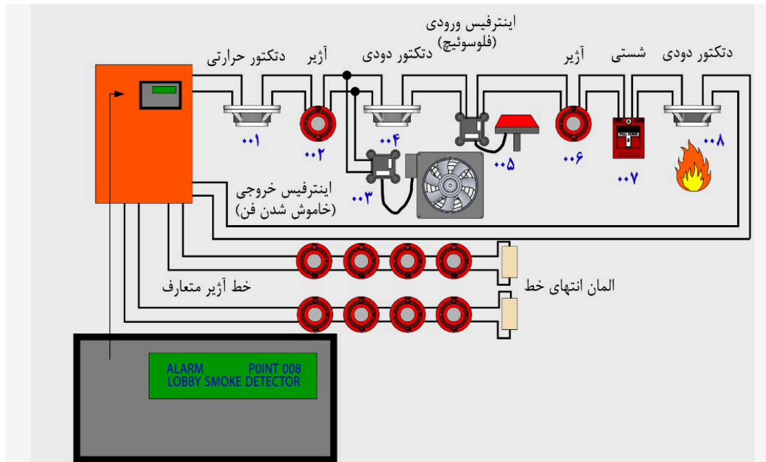
شکل ۴-۳- نمایش کابل‌کشی سیستم اعلام حریق آدرس‌پذیر و نمایش دتکتور فعال‌شده در صفحه نمایش
