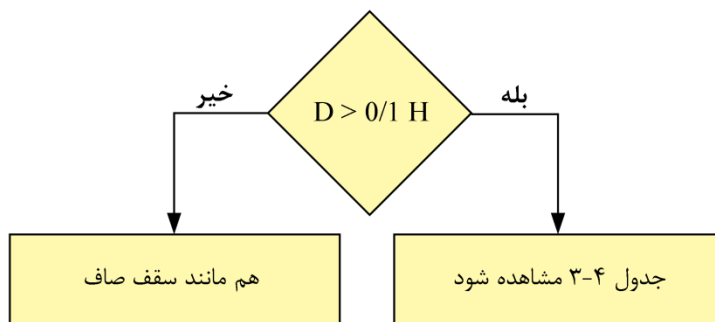
شکل ۴-۴۷- الزامات حدود فاصله و جانمایی دتکتور در سقف‌های دارای تیر یا تیرچه با فاصله نزدیک
