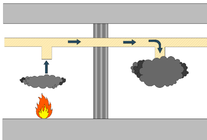
شکل ۴-۶۴- تصرفی بدون استفاده از دکتور کانالی - حریق توسط کانال سیستم تهویه به واحد (های) دیگر سرایت می کند.
