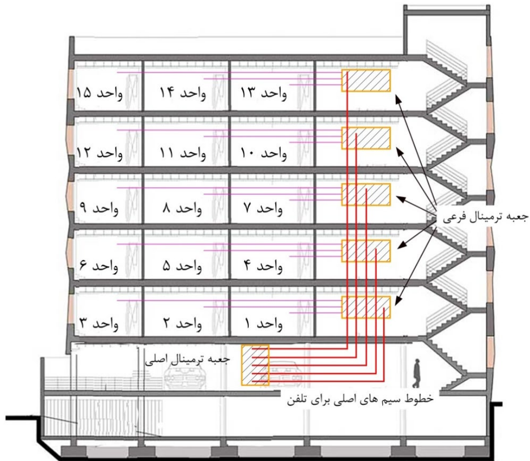
شکل ۱-۱۳- سیم‌کشی تلفن (روش اول)
