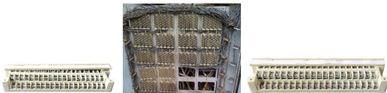
شکل ۱-۸- ترمینال‌های ۲۰، ۲۵ و ۱۰ زوجی پیچی
