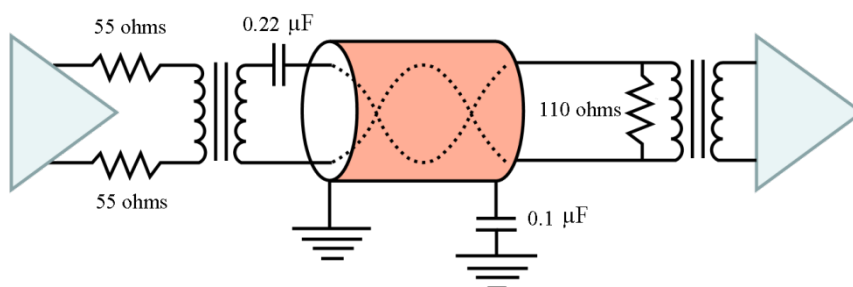
شکل ۷-۱۶- مبدل سیگنال متوازن
