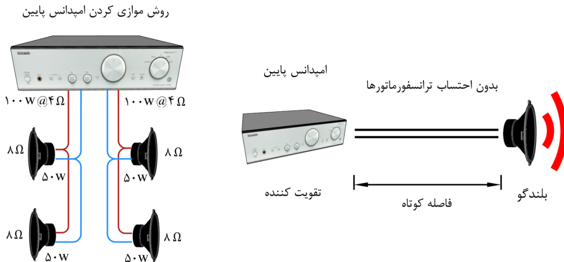
شکل ۷-۱۲۰- روش اتصال مستقیم بلندگوهای امپدانس پایین به تقویت‌کننده
