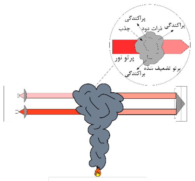
شکل ۴-۱۱- عملکرد دتکتور دودی خطی نوع منعکس کننده
