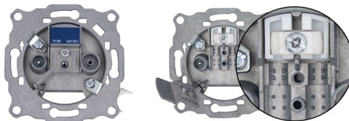
شکل ۲-۱۹- یک نمونه پریز میانی و نمای داخلی آن
