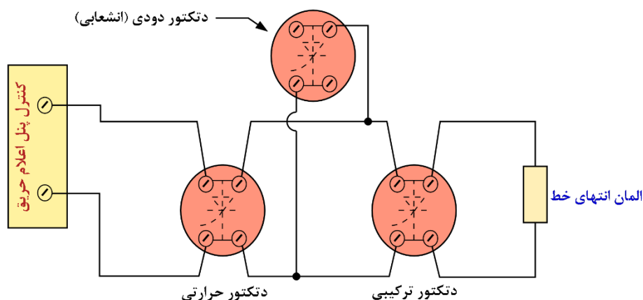
شکل ۴-۲- نمایش کابل کشی انشعاب T در سیستم کشف و اعلام حریق متعارف
