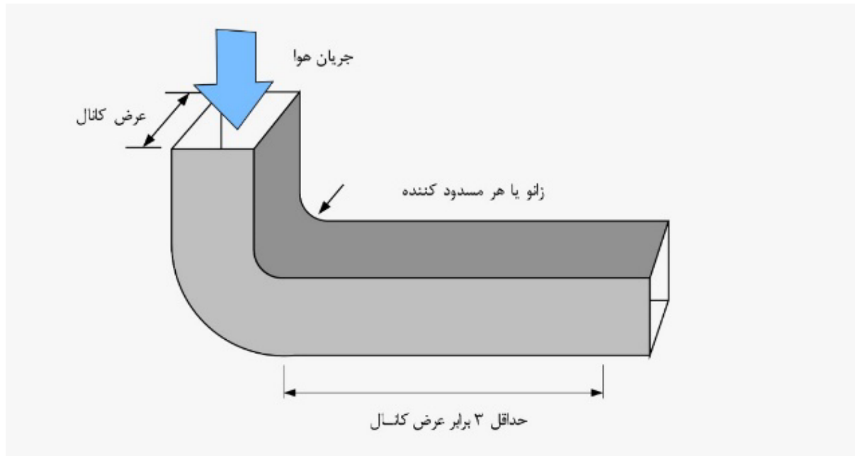
شکل ۴-۶۶- جانمایی صحیح دتکتور کانالی
