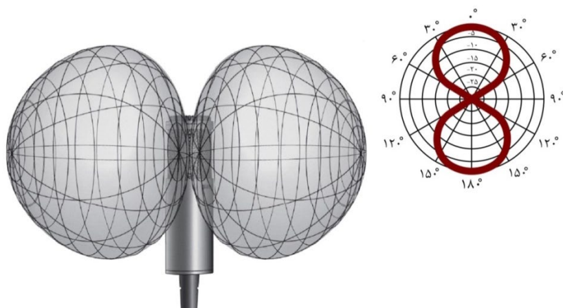
شکل ۷-۲۵ - منحنی و بالن الگوی دریافت میکروفن دو جهته یا الگوی ۸
