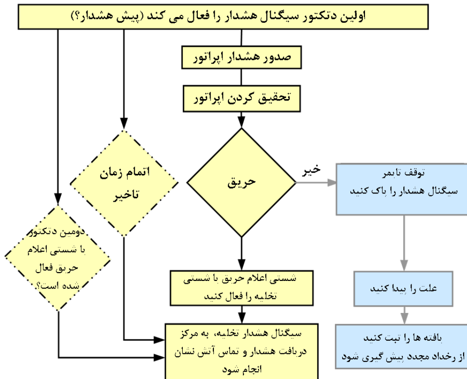
شکل ۴-۲۵- ترتیب هشدار اپراتور به صورت نمونه
