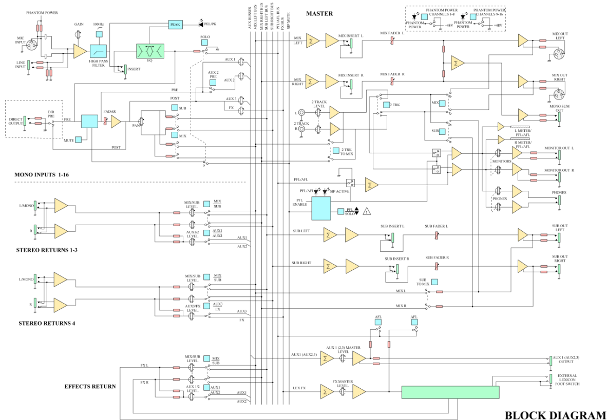
شکل ۷-۷۳ - یک نمونه بلوک دیاگرام میکسر صوتی
