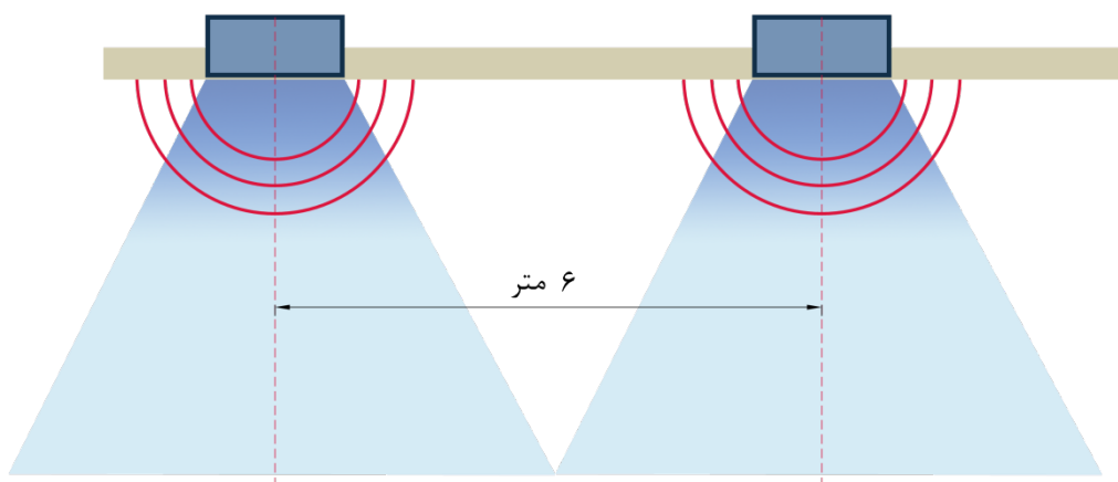
شکل ۵-۵- فاصله مجاز بین بلندگوهای سقفی
