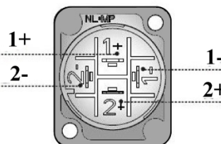
WIRING
