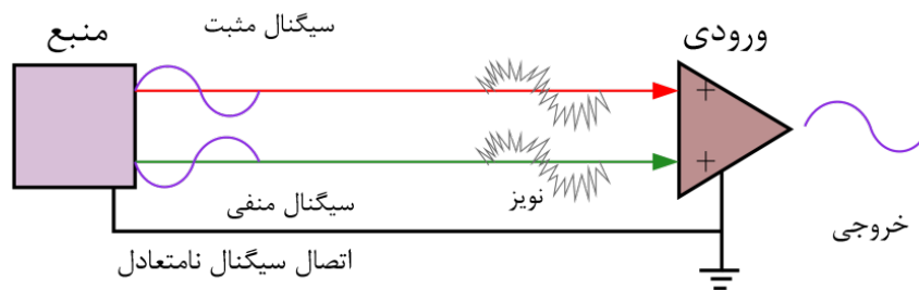
شکل ۷-۱۰- ارتباط منبع سیگنال با ورودی دستگاه به وسیله سیگنال متعادل
