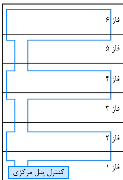
شکل ۴-۷۱- استفاده از کابل مقاوم در برابر حریق ارتقاء یافته در ساختمانی که دارای ۴ فاز تخلیه یا بیش‌تر است (بدون شبکه بارنده خودکار)
