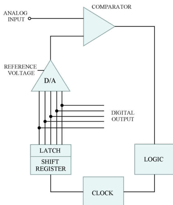
شکل ۷-۱۳- بلوک دیاگرام مبدل آنالوگ به دیجیتال تقریب متوالی
