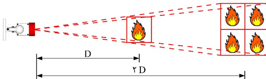
شکل ۴-۶۰- تاثیر افزایش فاصله منبع حریق از دتکتور شعله
