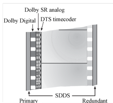
شکل ۷-۶۹- محل ضبط صدا با استانداردهای سینمایی بر روی فیلم ۳۵ میلی‌متری
