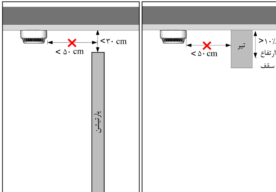
شکل ۴-۴۳- پارتیشن یا قفسه
