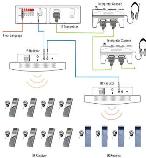
شکل ۸-۷- نحوه اتصالات یک سیستم ترجمه هم‌زمان دو زبانه
