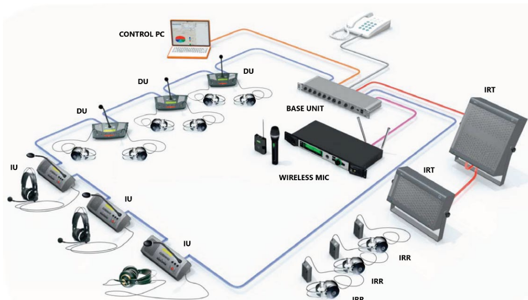
شکل ۸-۸ - نحوه اتصالات یک سیستم ترجمه هم‌زمان سه زبانه و سیستم کنفرانسی یک پارچه
