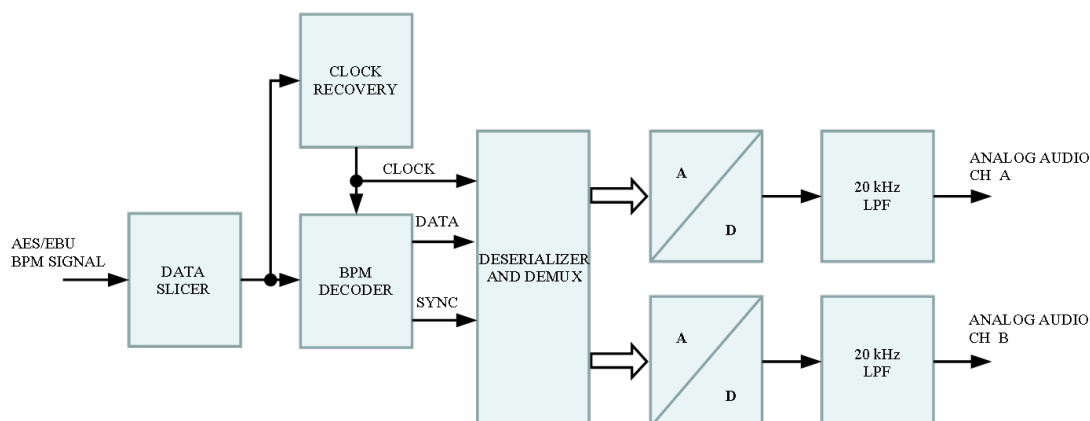
شکل ۷-۱۹- بلوک دیاگرام دکودر سیگنال دیجیتال AES/EBU
