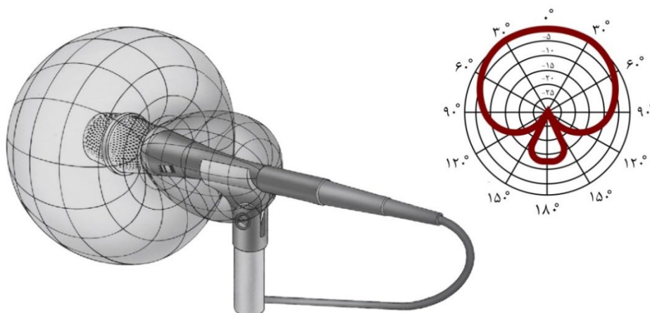
شکل ۷-۲۴ - منحنی و بالن الگوی دریافت میکروفن جهت‌دار با الگوی فوق‌العاده قلبی
