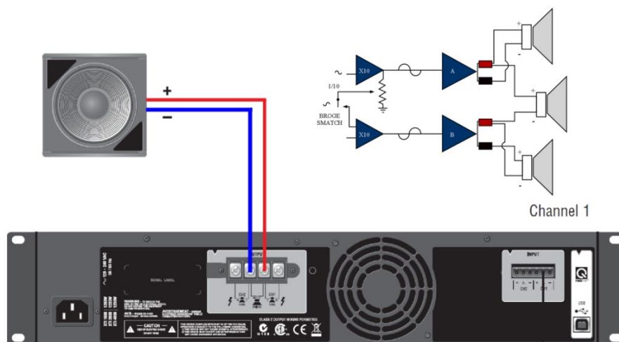
شکل ۷-۸۵- طریقه اتصال سیگنال و بلندگو به تقویت کننده در حالت بریج
