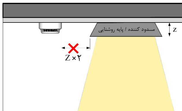
شکل ۴-۴۲- رعایت فاصله مجاز جهت جانمایی دتکتور از موانع جریان دود
