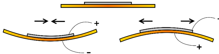
شکل ۷-۱۱۲- طرز کار یک قطعه پیزوالکتریک
