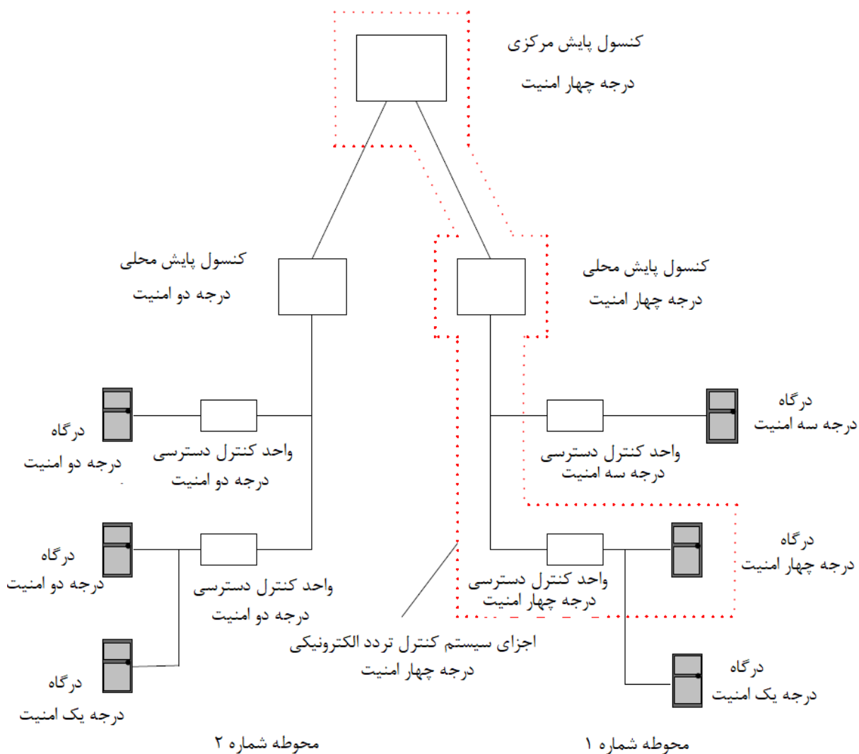
شکل ۳-۳۱- مثالی از انتخاب درجه امنیت در سیستم کنترل دسترسی الکترونیکی
