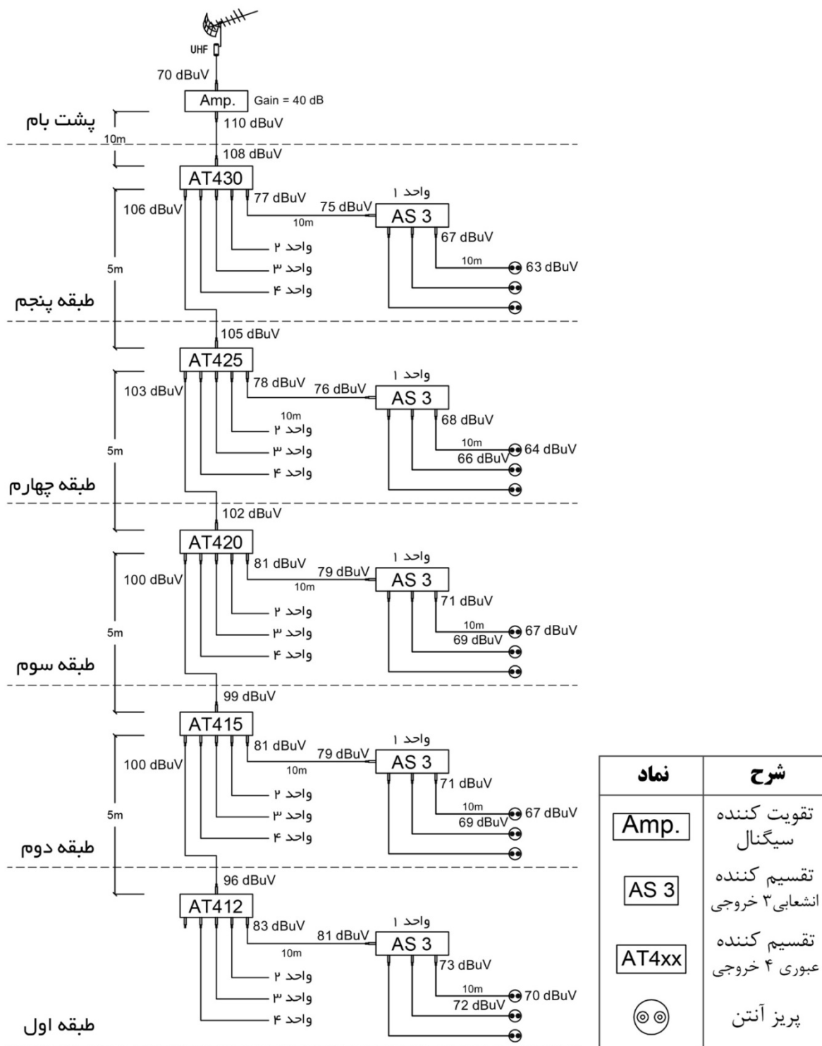
شکل ۲-۲۵- یک نمونه فرضی دیاگرام آنتن مرکزی و اجزای تشکیل دهنده آن به همراه محاسبات
