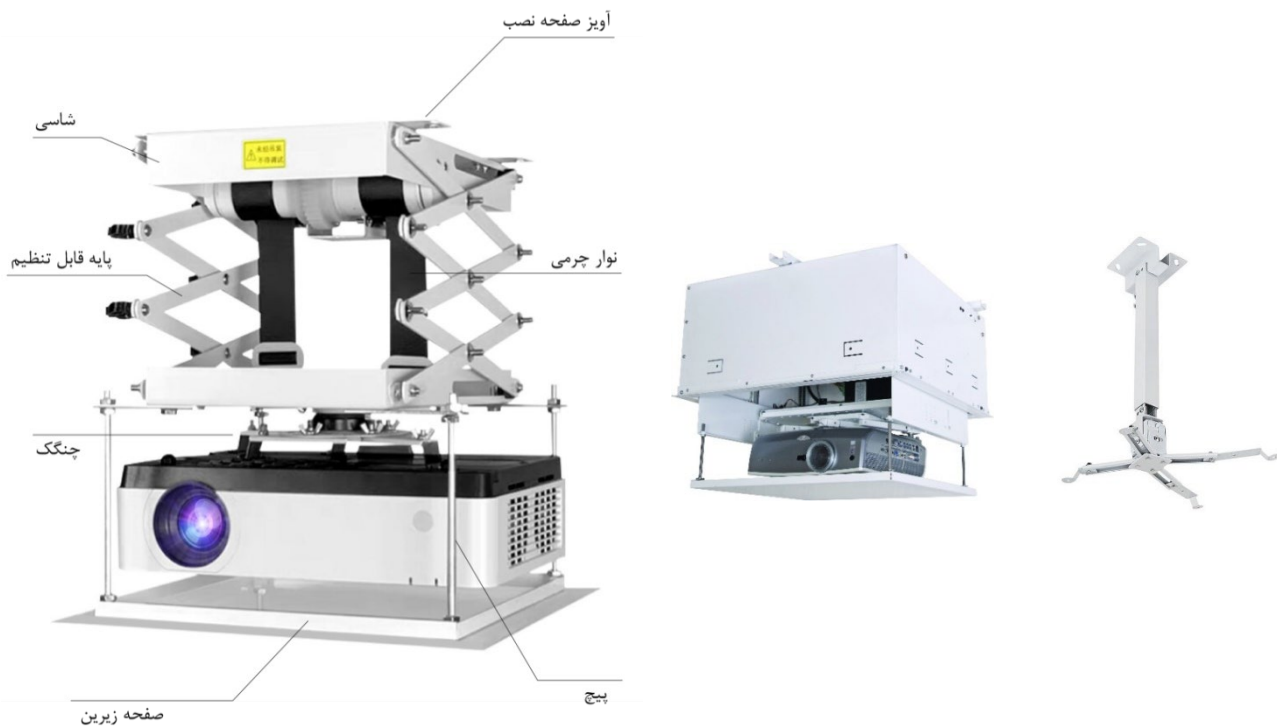
دو نمونه پایه ویدیو پروژکتور متحرک برقی
