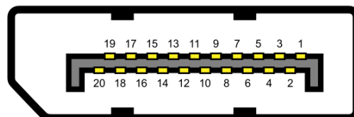
شکل ۸-۳۰- شماره پایه‌های سوکت DP
