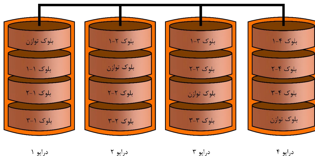
شکل ۳-۲۱- استفاده از تکنولوژی ذخیره‌ساز پشتیبان مستقل ۱ جهت افزایش امنیت اطلاعات
