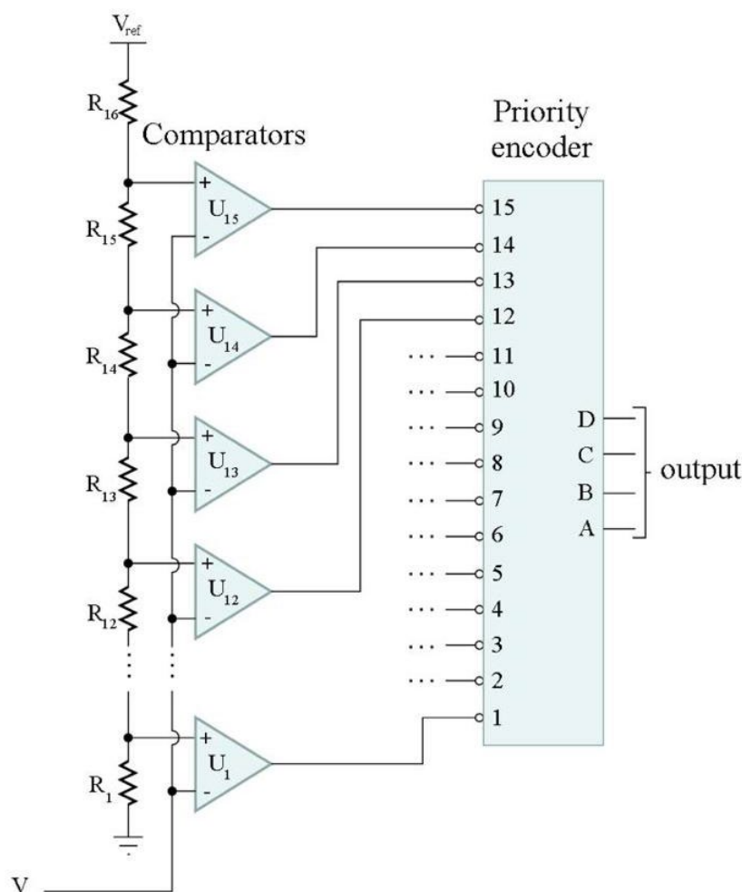
شکل ۷-۱۲- بلوک دیاگرام مبدل آنالوگ به دیجیتال فلش
