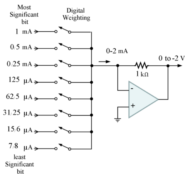
شکل ۷-۱۵- نمونه ساده شده مبدل متعارف نردبانی
