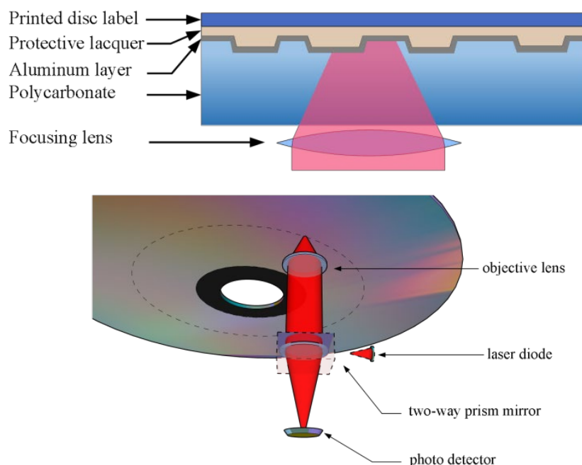
شکل ۷-۹۸- ساختار دیسک و خواندن اطلاعات یک دیسک
