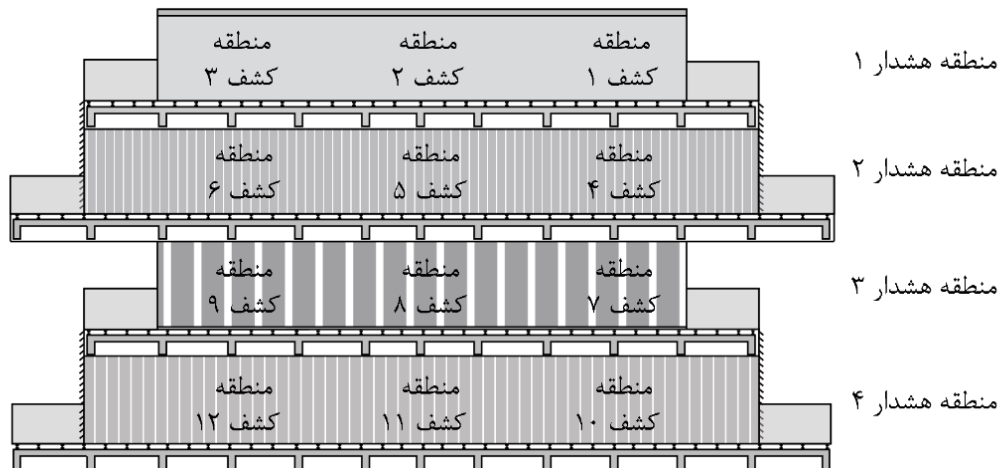
شکل ۴-۲۳- منطقه هشدار با چندین منطقه کشف
