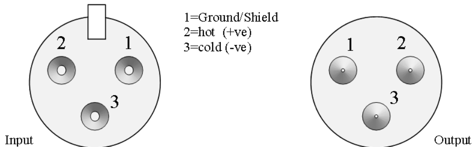
شکل ۷-۱۴۳- ترتیب اتصال پایه‌ها به سیگنال متوازن
