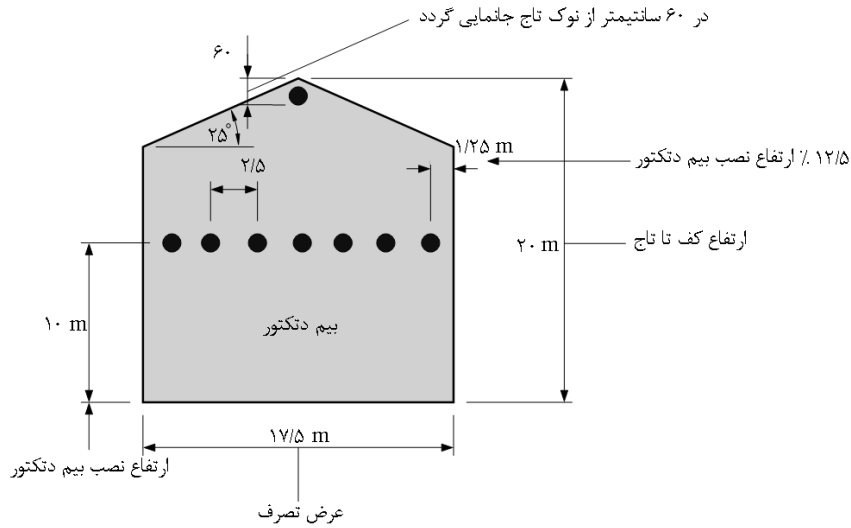
شکل ۴-۵۵- جانمایی دتکتور دودی خطی (بیم دتکتور)
