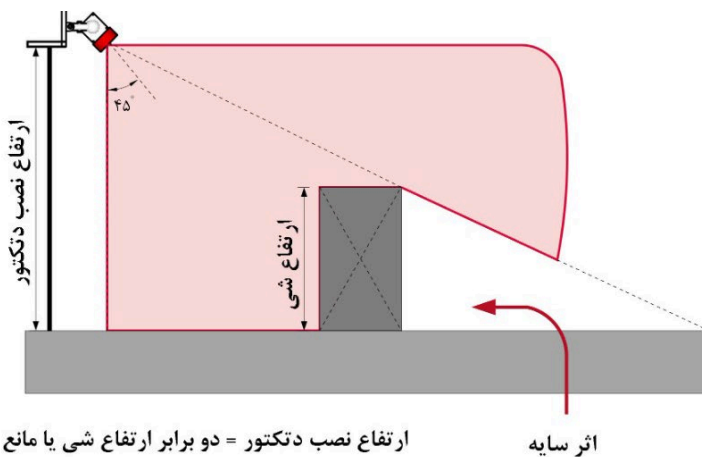
شکل ۴-۶۱- اثر سایه
