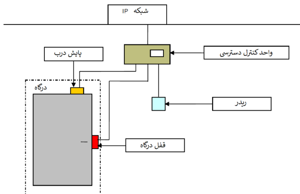
شکل ۳-۳۰- شمای کلی از یک درگاه مجهز به سیستم کنترل دسترسی الکترونیکی تحت شبکه
