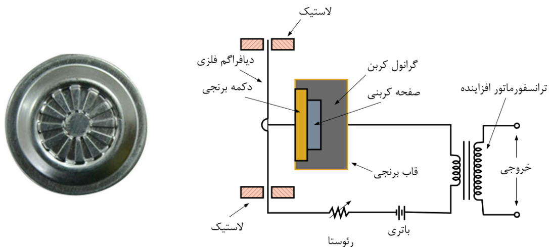
شکل ۷-۲۹ - ساختمان داخلی و یک نمونه کپسول میکروفن کربنی
