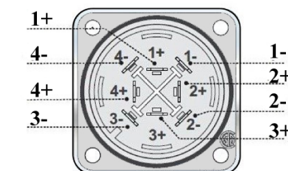
WIRING
