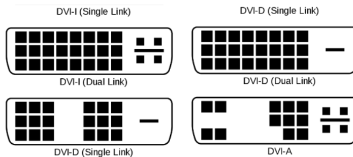
شکل ۸-۲۴- پایه‌های مختلف چند نمونه سوکت DVI
