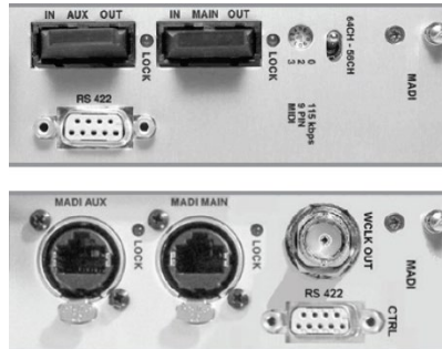
شکل ۷-۲۰ - دو نمونه کارت ارتباطی MADI
