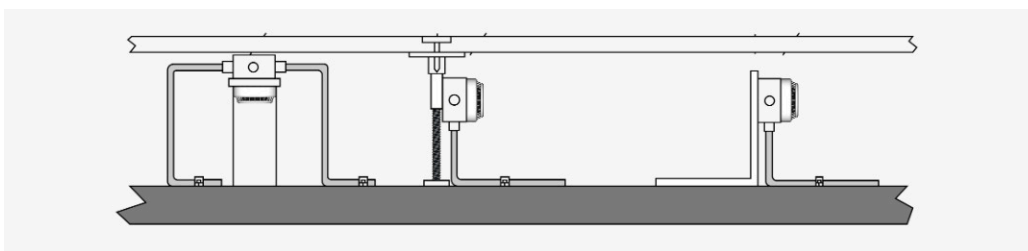
شکل ۴-۳۲- نصب صحیح دکتور در کف کاذب
