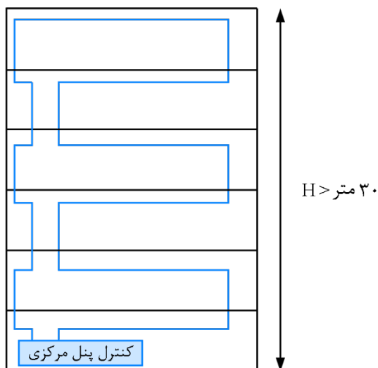
شکل ۴-۷۲- استفاده از کابل مقاوم در برابر حریق ارتفاع یافته در ساختمانی با ارتفاع بیش از ۳۰ متر (بدون شبکه بارنده خودکار)
