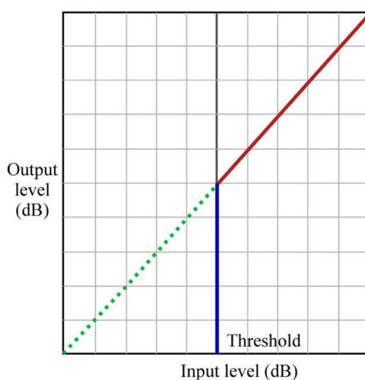
شکل ۷-۵۴- منحنی تابع دستگاه گیت
