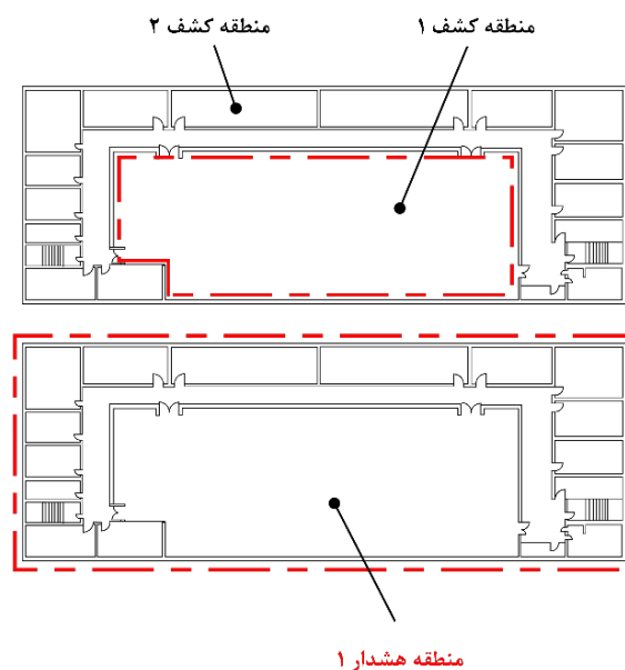
شکل ۴-۱۹- منطقه هشدار
