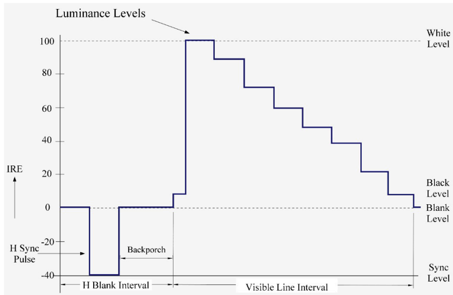
شکل ۸-۱۶- نمونه منحنی سیگنال تصویر سیاه و سفید
