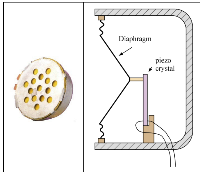
شکل ۷-۲۸ - ساختمان داخلی و یک نمونه کپسول میکروفن سرامیکی
