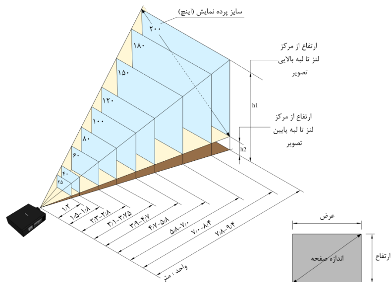
شکل ۸-۳۴- یک نمونه فاصله ویدیو پروژکتور متناسب با ابعاد پرده
