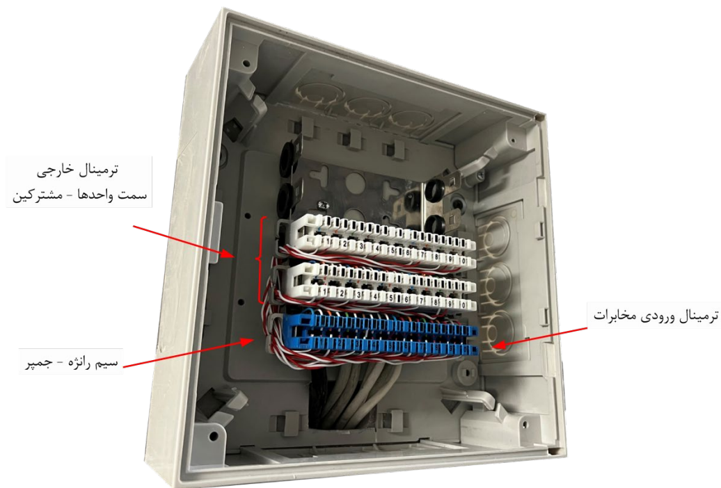
شکل ۱-۱- جعبه ترمینال اصلی تلفن
