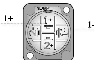
WIRING
