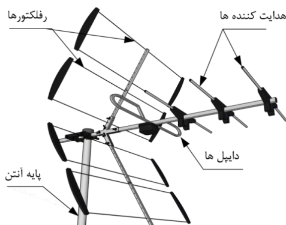
شکل ۲-۵ - اجزا تشکیل دهنده آنتن UHF
