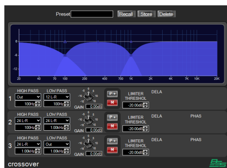
شکل ۷-۶۱- نمونه نرم‌افزار کنترل کراس‌اُور دیجیتال
