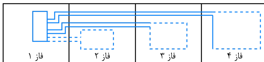
شکل ۴-۷۳- یک مثال از عبور کابل‌های سیگنال حیاتی مرتبط با مناطق دور از حریق
