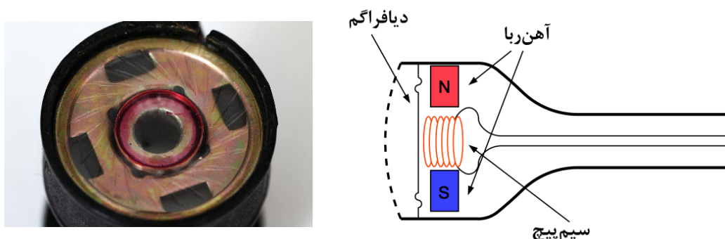
شکل ۷-۲۶- ساختمان داخلی و یک نمونه کپسول میکروفن داینامیک
