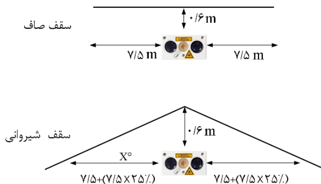
شکل ۴-۵۴- پوشش دهی دکتور دودی خطی در سقف‌های صاف و شیب‌دار
