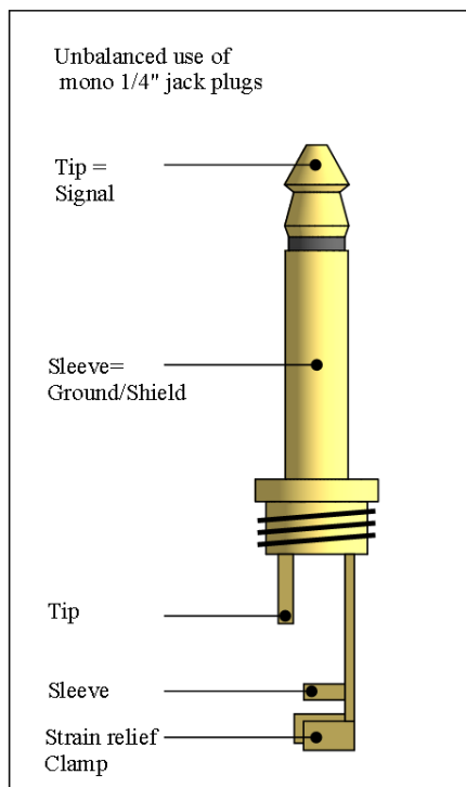
شکل ۷-۱۴۷- یک نمونه فیش TS و نام‌گذاری و اتصال پایه‌های آن
