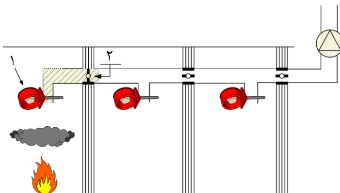
شکل ۴-۶۴- تصرفی بدون استفاده از دکتور کانالی - حریق توسط کانال سیستم تهویه به واحد (های) دیگر سرایت می کند.
