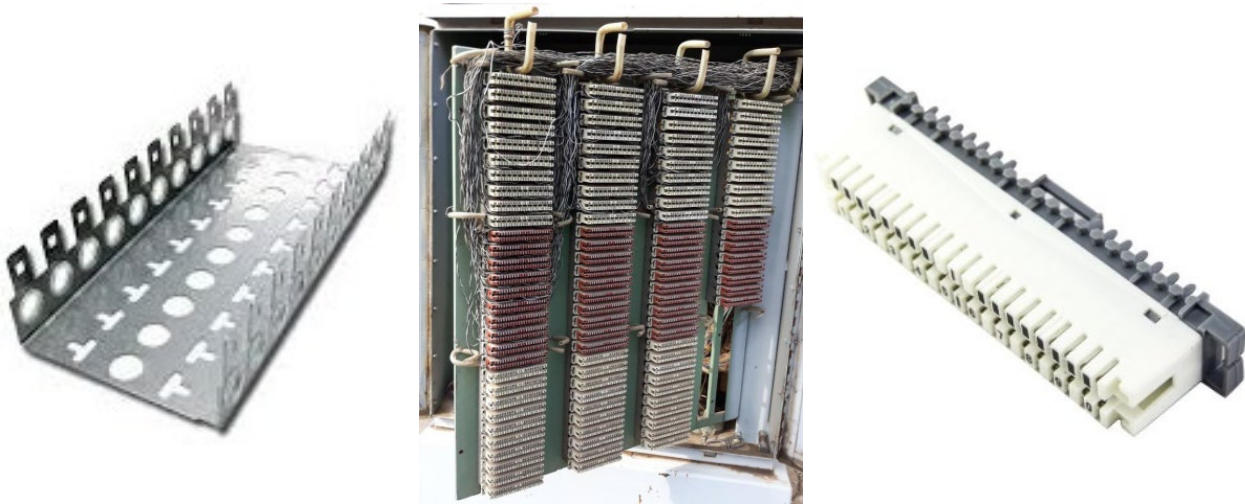
شکل ۱-۹- ترمینال ۱۰ زوجی، دسته‌های ۱۰۰ تایی و پایه ترمینال کروم
