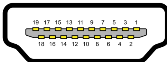
شکل ۲۸-۸- شماره پایه‌های کانکتورهای HDMI
