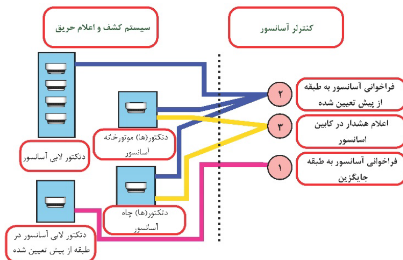
شکل ۴-۷۶- سناریو حریق در آسانسور
