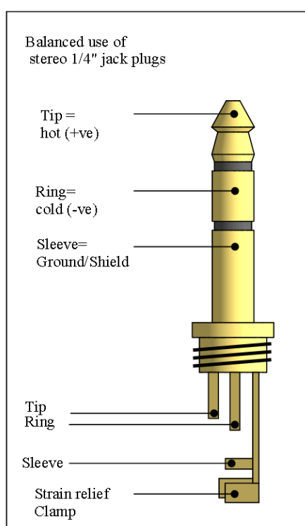
شکل ۷-۱۴۵- نام‌گذاری و اتصال پایه‌ها در فیش TRS
