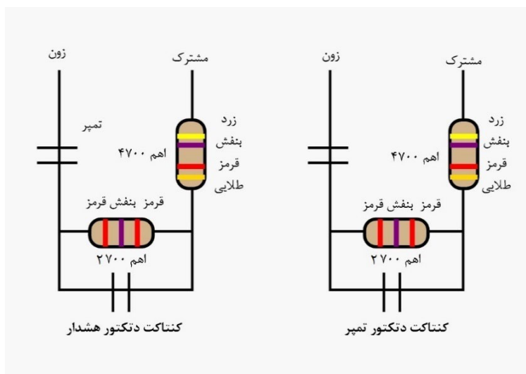
شکل ۳-۱۰- نحوه ارتباط دکتورها با مرکز کنترل سیستم هشدار در درجه امنیت سه
