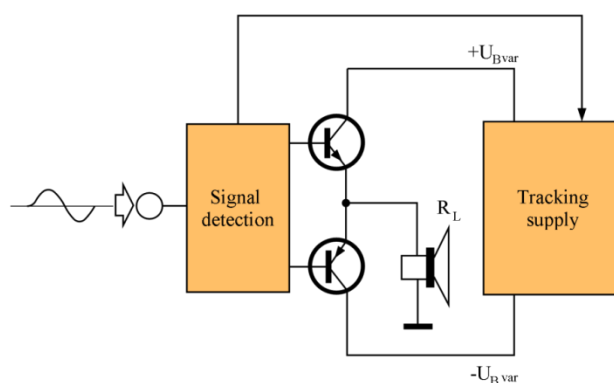
شکل ۷-۹۵- بلوک دیاگرام مدار تقویت‌کننده کلاس G
