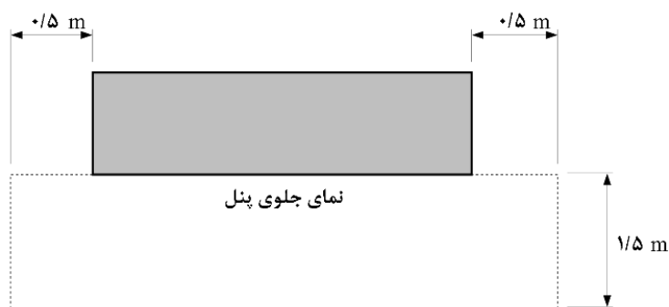
شکل ۴-۶۹- حریم کنترل پنل
