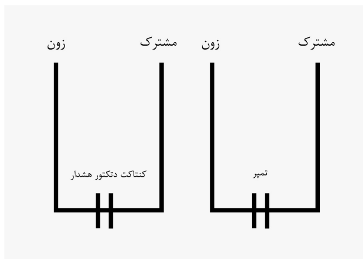
شکل ۳-۹- نحوه ارتباط دتکتورها با مرکز کنترل سیستم هشدار در درجه امنیت دو
