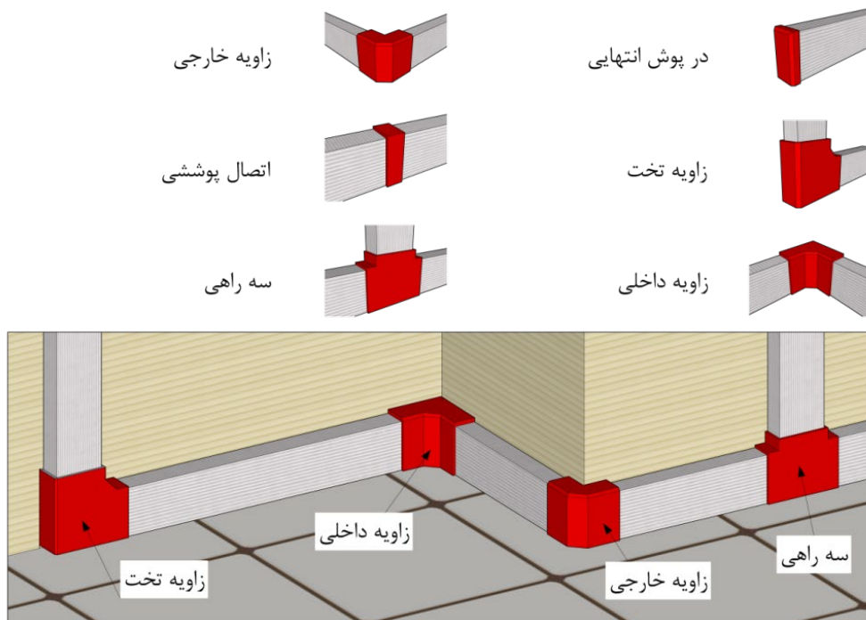
شکل ۱-۱۴ - شماتیک (الف): نحوه نصب تجهیزات. شماتیک (ب): محل قرار گیری آن‌ها.
