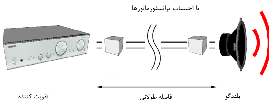
شکل ۷-۱۲۱- روش اتصال بلندگوهای امپدانس بالا از طریق ترانسفورماتور تطبیق امپدانس به تقویت‌کننده
