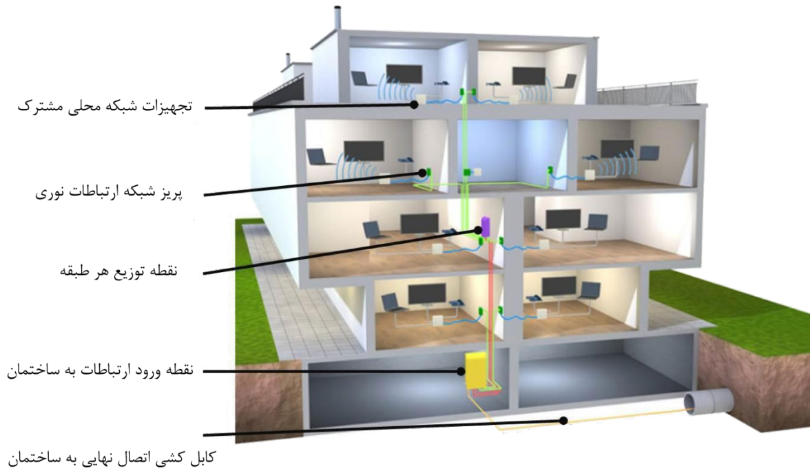
شکل ۱۵-۱- شماتیک ارتباطات نوری و تجهیزات ورودی و داخل ساختمان
