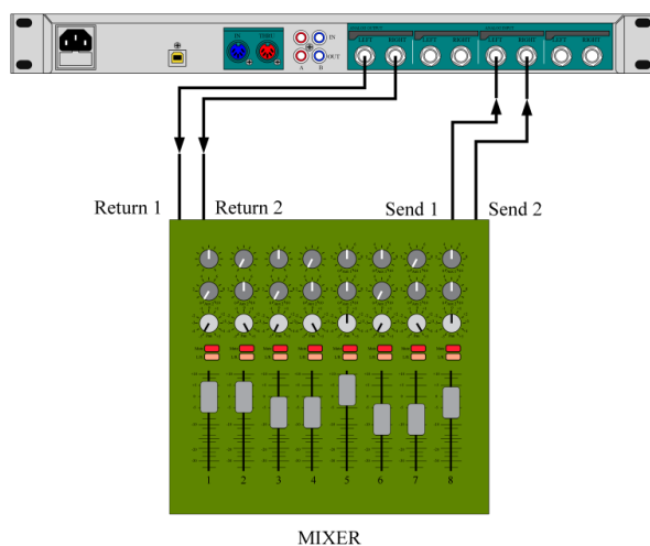
شکل ۷-۶۷- بلوک دیاگرام اتصال افکت پروسسور به میکسر صوتی
