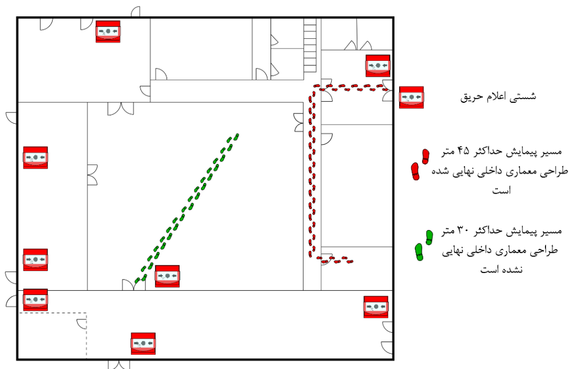
شکل ۴-۲۷- حداکثر پیمایش جهت فعال‌سازی شستی اعلام حریق
