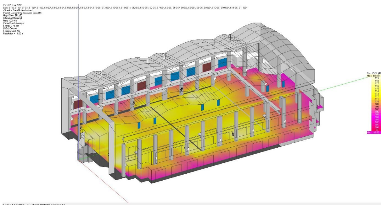
شکل ۷-۱۵۹- یک نمونه خروجی نرم افزار آکوستیک
