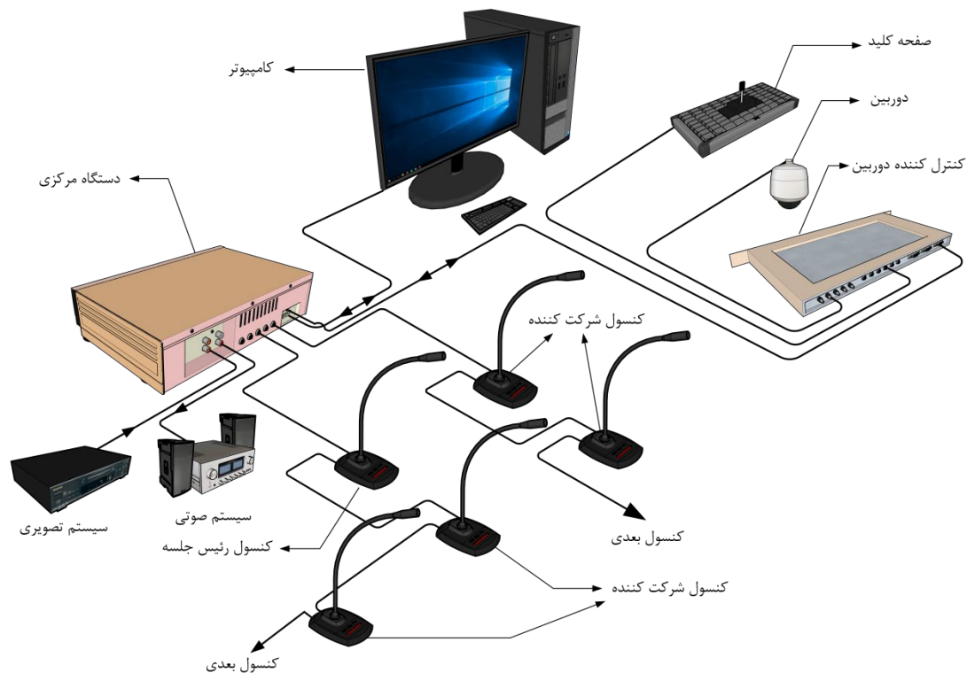
شکل ۸-۴۲- بلوک دیاگرام و اتصالات اجزاء یک سیستم کنفرانسی با تجهیزات دنبال کننده تصویری
