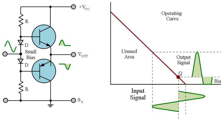
شکل ۷-۹۲- یک نمونه مدار ساده و منحنی نقطه کار و خط بار تقویت‌کننده کلاس AB
