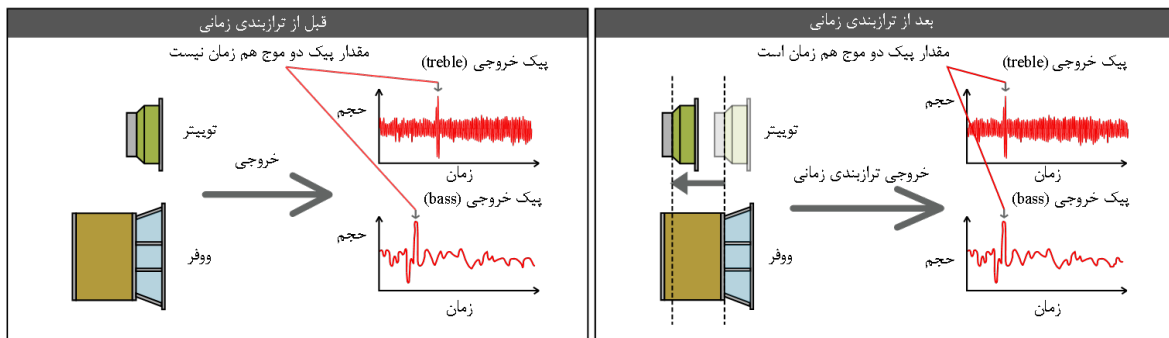
شکل ۷-۴- ساختار و صدای خروجی دو بلندگو با واحد راه‌اندازهای با فاصله و واحد راه‌اندازهای هم تراز
