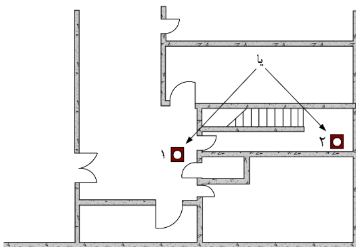
شکل ۴-۲۶- جانمایی شستی اعلام حریق در مسیرهای فرار - شستی اعلام حریق می‌تواند در موقعیت ۱ یا ۲ جانمایی شود.
