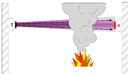
شکل ۴-۱۰- عملکرد دتکتور دودی خطی نوع فرستنده - گیرنده
