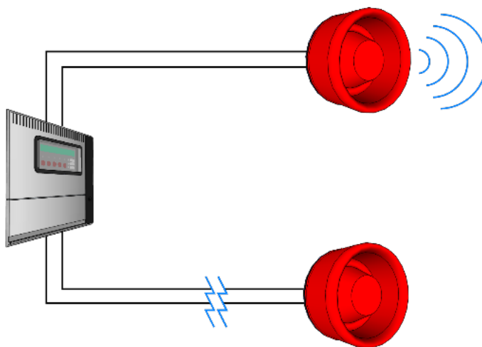
شکل ۴-۷۴- توزیع آژیر در سیستم اعلام حریق متعارف
