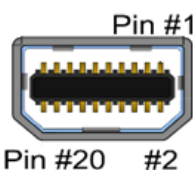
شکل ۸-۳۲- پایه‌های سوکت mini DP
