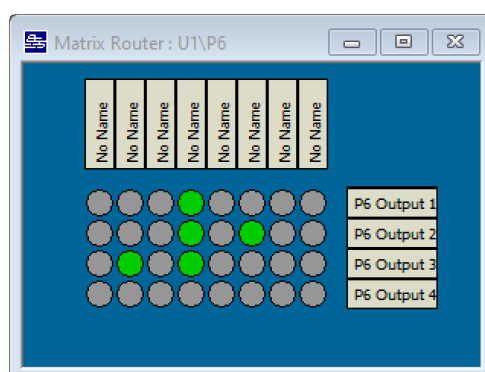
شکل ۷-۵۸ - نمونه نرم‌افزار کنترل ماتریس صوتی دیجیتال
