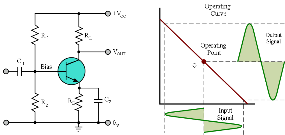
شکل ۷-۹۰- یک نمونه مدار ساده و منحنی نقطه کار و خط بار تقویت‌کننده کلاس A
