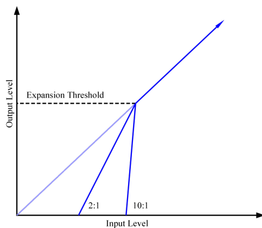
شکل ۷-۵۵- منحنی تابع دستگاه اکسپندر
