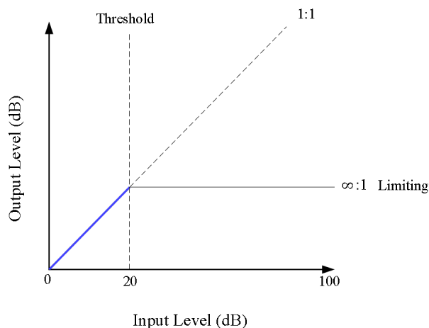
شکل ۷-۴۹ - منحنی تابع دستگاه لیمیتر
