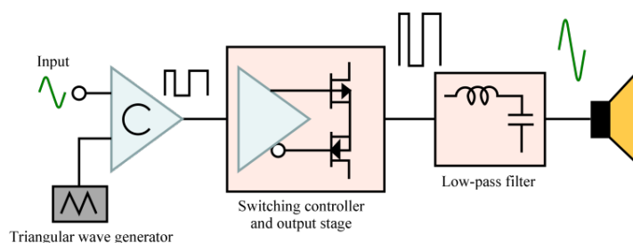
شکل ۷-۹۴- بلوک دیاگرام مدار تقویت‌کننده کلاس D
