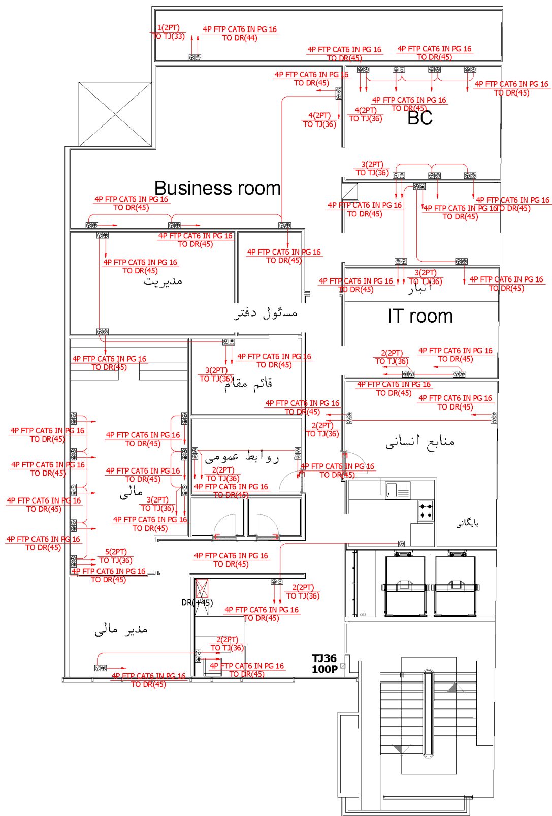
شکل ۱-۱۲- نقشه تلفن و شبکه یک مجموعه اداری
