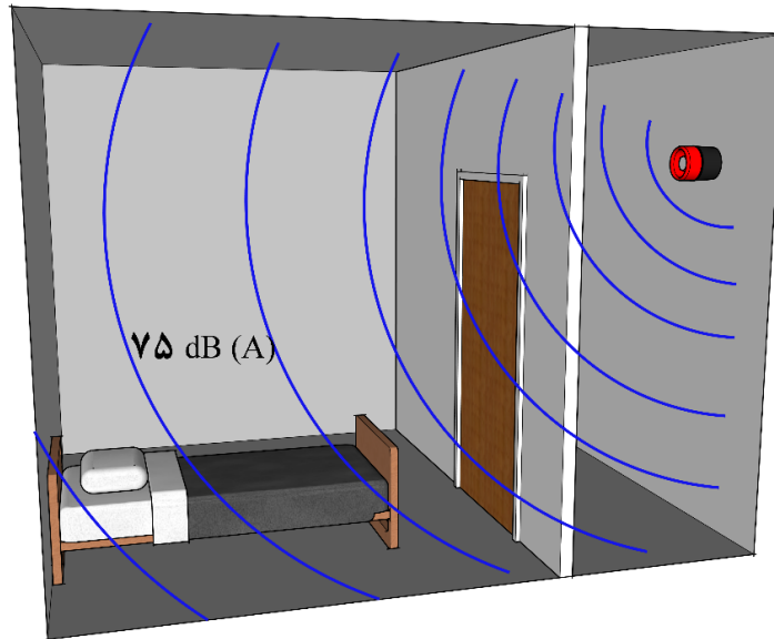
شکل ۴-۲۱- حداقل شدت صوت آژیر در فضاهای خوابیدن
