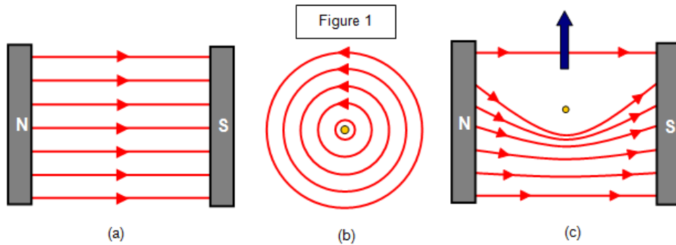
شکل ۷-۱۰۸- انرژی مکانیکی حاصل از سیم حامل جریان در میدان مغناطیسی
