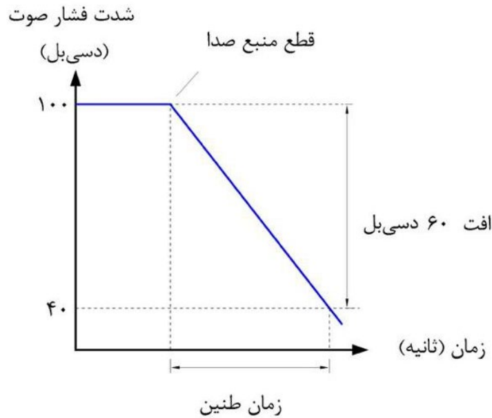
شکل ۷-۷- منحنی زمان RT_{60}
