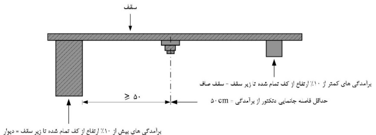
شکل ۴-۴۴- موانع موجود در سقف
