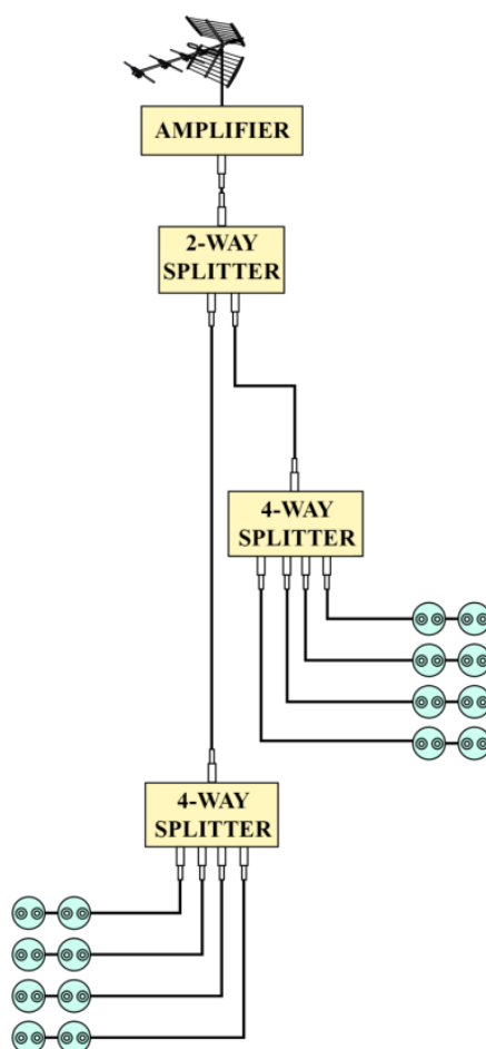
شکل ۲-۲۳- نمونه‌ای از دیاگرام آنتن مرکزی و اجزا تشکیل‌دهنده آن در روش اول
