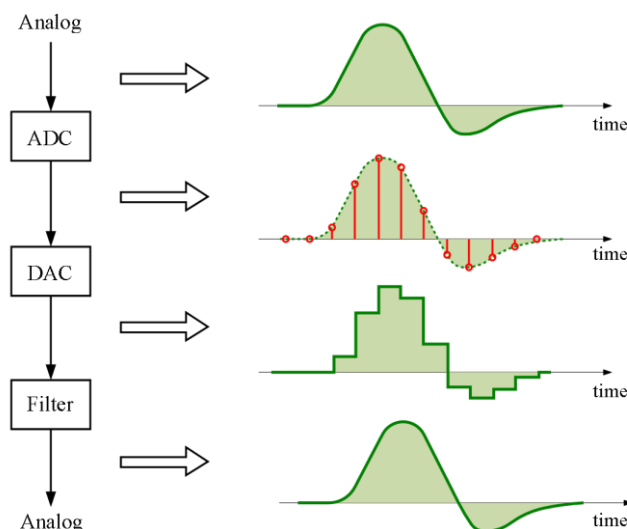
شکل ۷-۱۱- روش نمونه برداری و تبدیل سیگنال آنالوگ به دیجیتال و دیجیتال به آنالوگ
