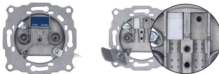
شکل ۲-۲۰- یک نمونه پریز انتهایی و نمای داخلی آن
