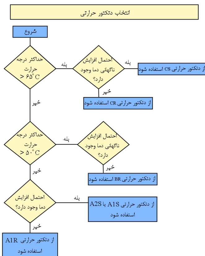
شکل ۴-۵۳- راهنمای انتخاب نوع و کلاس دتکتور حرارتی
