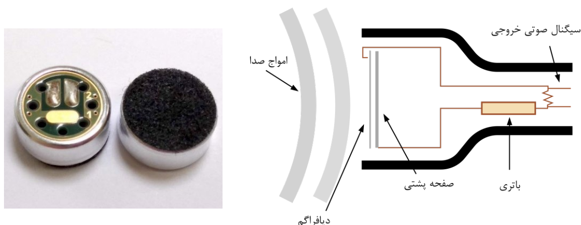
شکل ۲۷-۷- ساختمان داخلی و یک نمونه کپسول میکروفن خازنی
