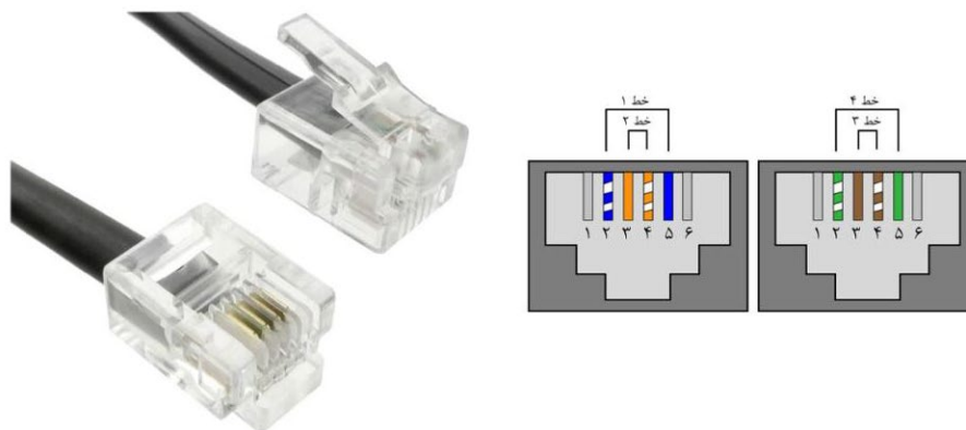
شکل ۱-۳- فیش تلفن RJ11
