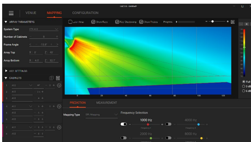
شکل ۷-۱۲۹- یک نمونه نرم‌افزار طراحی و آنالیز بلندگوهای آرایه‌ای خطی
