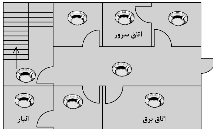
شکل ۴-۱۵- سیستم رسته حفاظت از اموال
