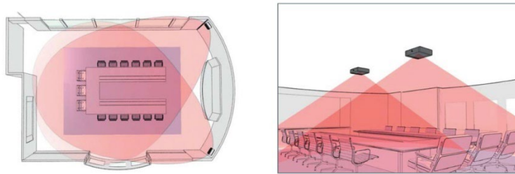
شکل ۸-۱۳- نمونه الگوی پخش نور تشعشع‌کننده مادون قرمز
