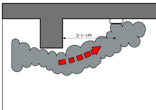
شکل ۴-۴۱- رعایت فاصله مجاز جهت جانمایی دتکتور از موانع جریان دود، گازهای داغ و دیوار
