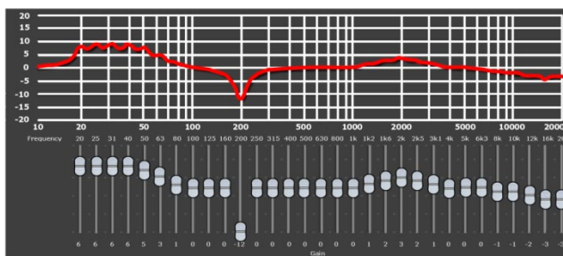
شکل ۷-۴۵- نمونه نرم‌افزار کنترل گرافیک اکولایزر دیجیتال و منحنی پاسخ فرکانسی آن
