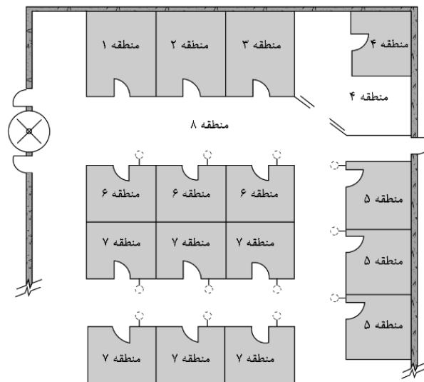
شکل ۴-۱۸- الف- نمونه تخصیص منطقه کشف برای مناطق مجاور و غیر همجوار
