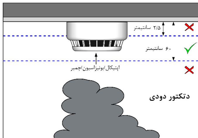
شکل ۴-۳۸- محدوده مجاز دکتور دودی
