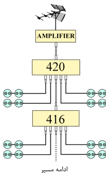
شکل ۲-۲۴- نمونه‌ای از دیاگرام آنتن مرکزی و اجزا تشکیل‌دهنده آن در روش دوم
