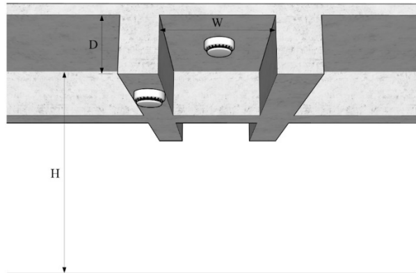
شکل ۴-۴۵- سقف افقی شامل سلول‌های کوچک
