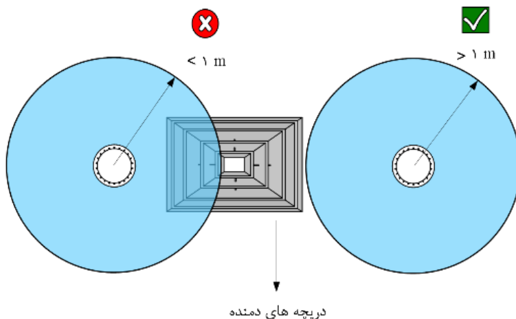
شکل ۴-۵۱- رعایت فاصله جانمایی مجاز دکتور از دریچه دمنده
