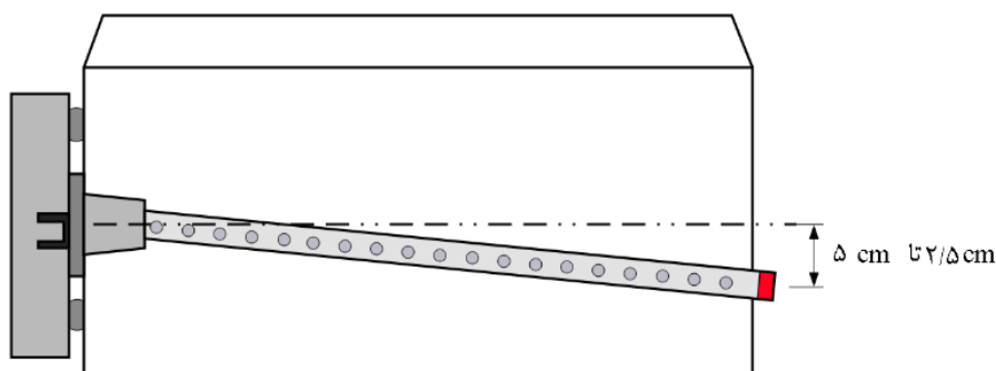
شکل ۴-۶۸- نصب صحیح دتکتور کانالی
