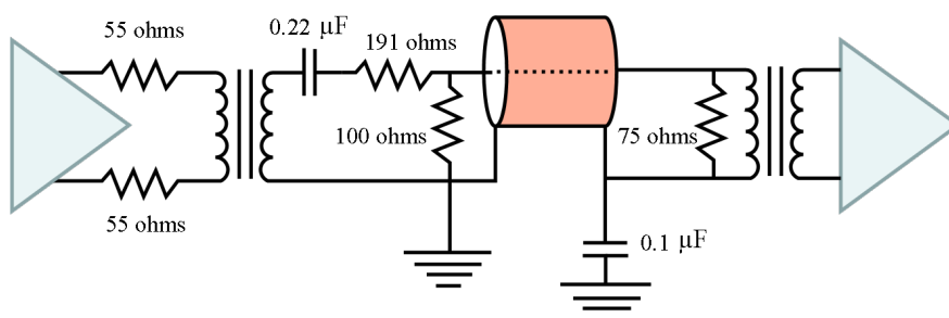
شکل ۷-۱۷- مبدل سیگنال نامتوازن
