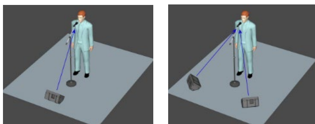
شکل ۷-۱۳۸- روش استفاده از یک یا دو بلندگوی مانیتور سن
