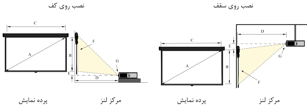
شکل ۸-۳۳- یک نمونه ابعاد مختلف پرده و فاصله ویدیو پروژکتور
