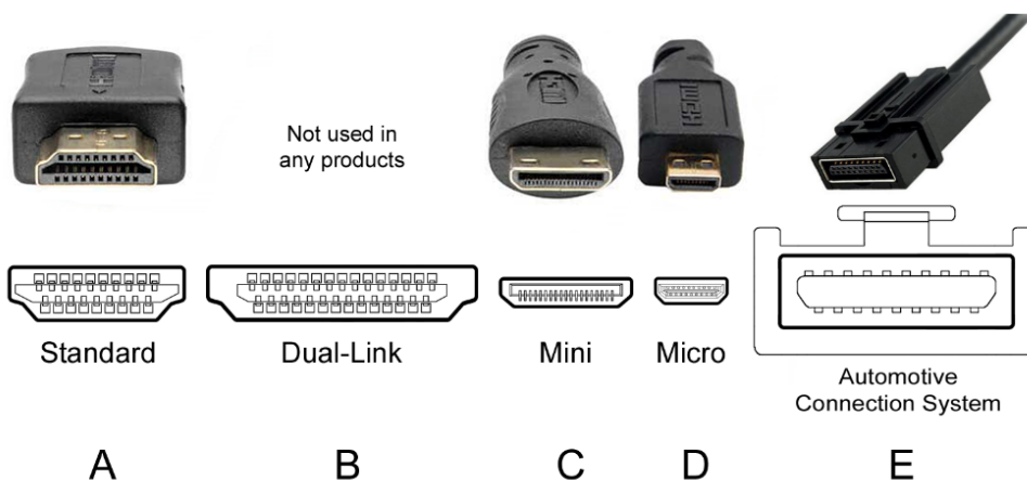
شکل ۲۷-۸- انواع مختلف کانکتورهای HDMI
