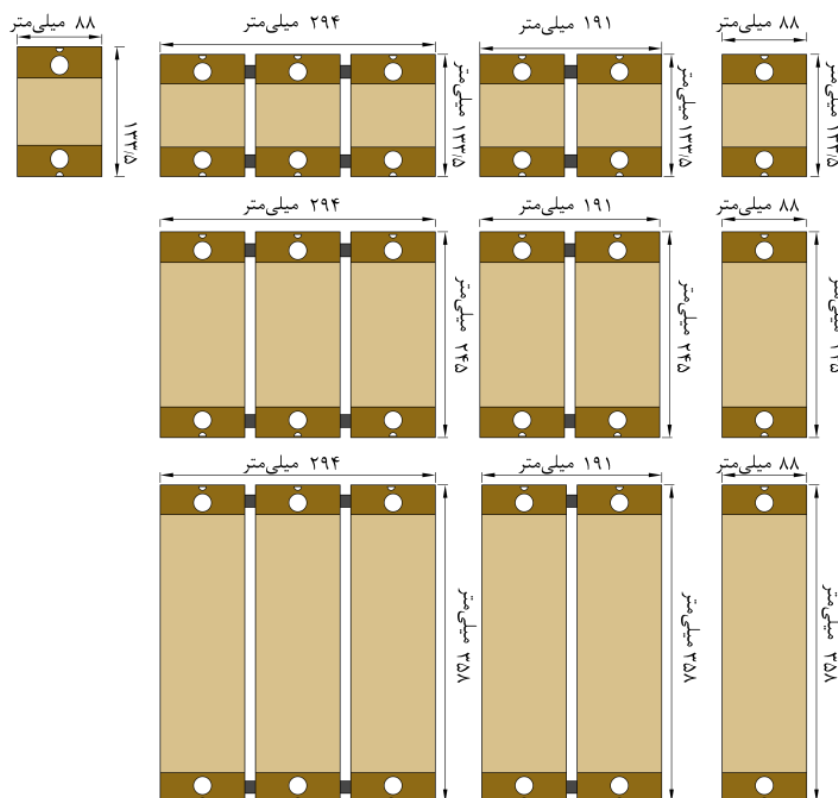
شکل ۶-۴- نمونه‌ای از قوطی‌های توکار پنل
