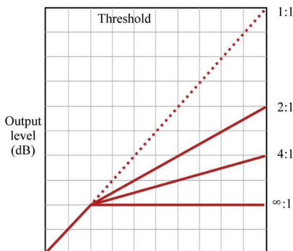
شکل ۷-۵۱ - منحنی تابع دستگاه کمپرسور
