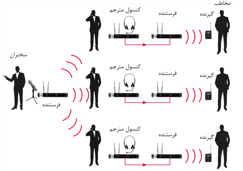
شکل ۸-۶- بلوک دیاگرام یک نمونه سیستم ترجمه هم‌زمان سه زبانه
