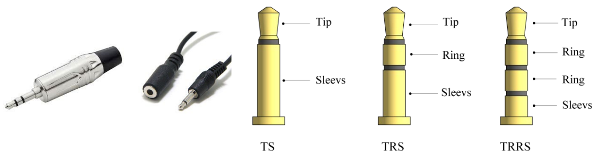
شکل ۷-۱۴۸- دو نمونه جک مادگی و فیش نری ۲٫۵mm
