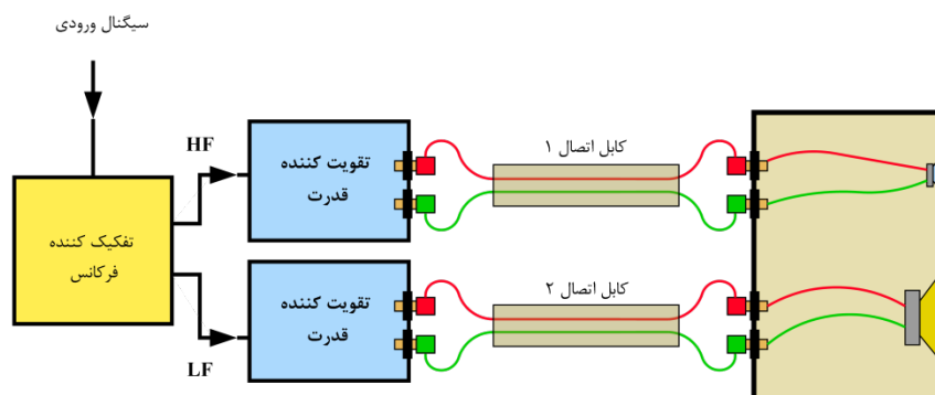
شکل ۷-۶۰- بلوک دیاگرام اتصال یک تفکیک‌کننده فرکانسی فعال و تقویت‌کننده و بلندگوی بای‌امپ
