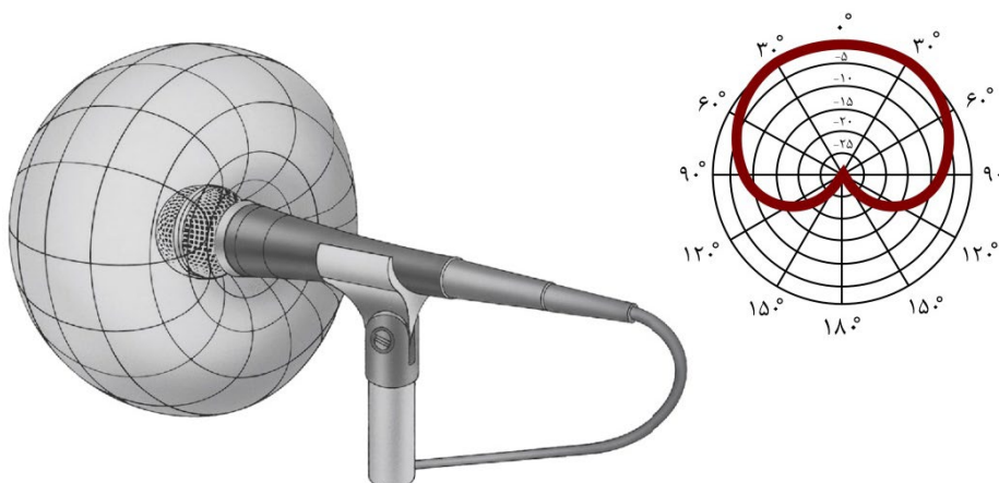
شکل ۷-۲۳- منحنی و بالن الگوی دریافت میکروفن جهت دار با الگوی قلبی
