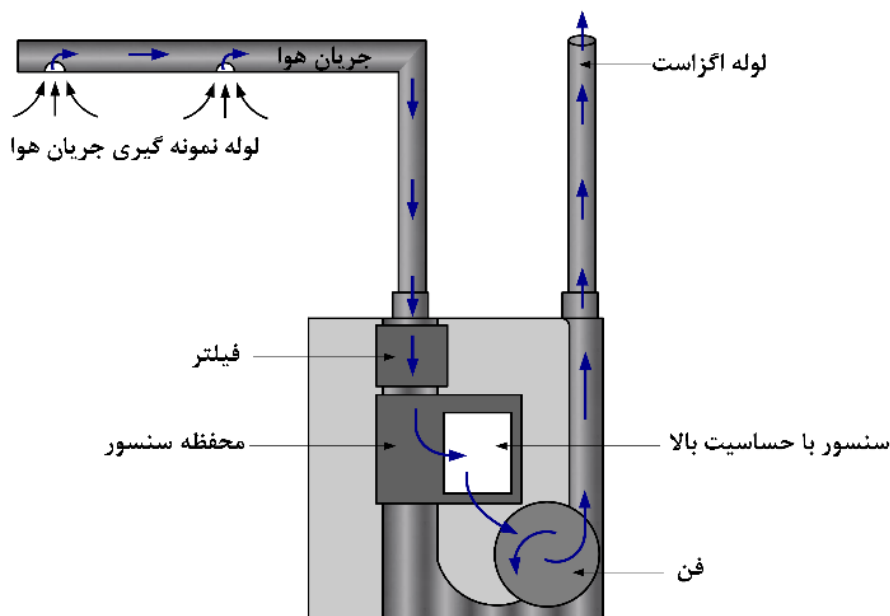
شکل ۴-۶- دتکتور مکنده دودی
