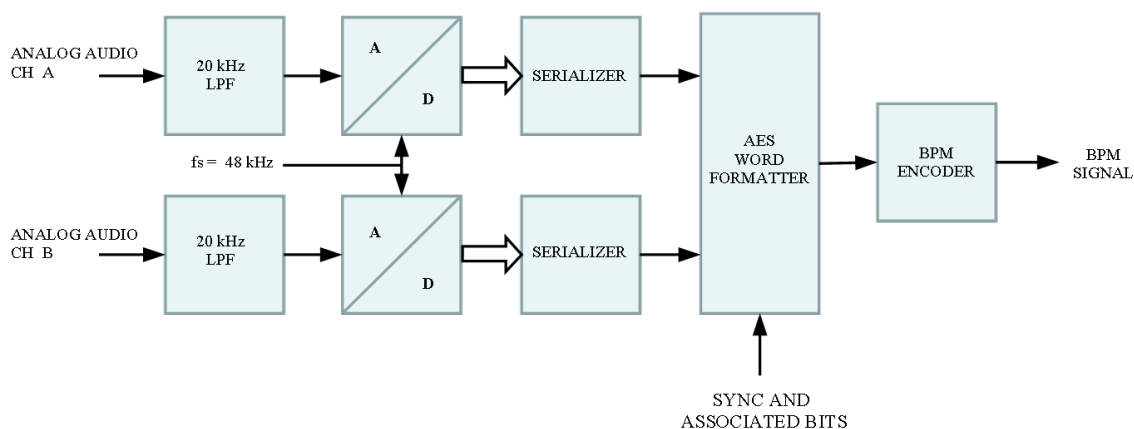
شکل ۷-۱۸- بلوک دیاگرام انکودر سیگنال دیجیتال AES/EBU
