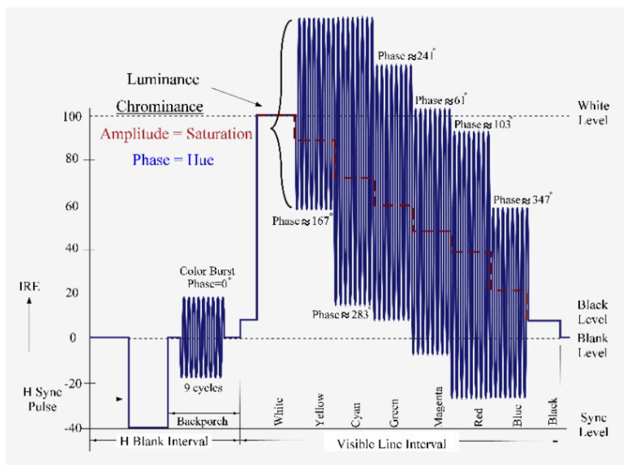
شکل ۸-۱۷- نمونه شکل موج سیگنال ویدئو رنگی
