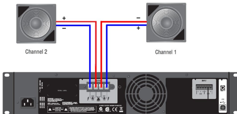
شکل ۷-۸۴- طریقه اتصال تقویت‌کننده به بلندگو در حالت دوتایی و Y
