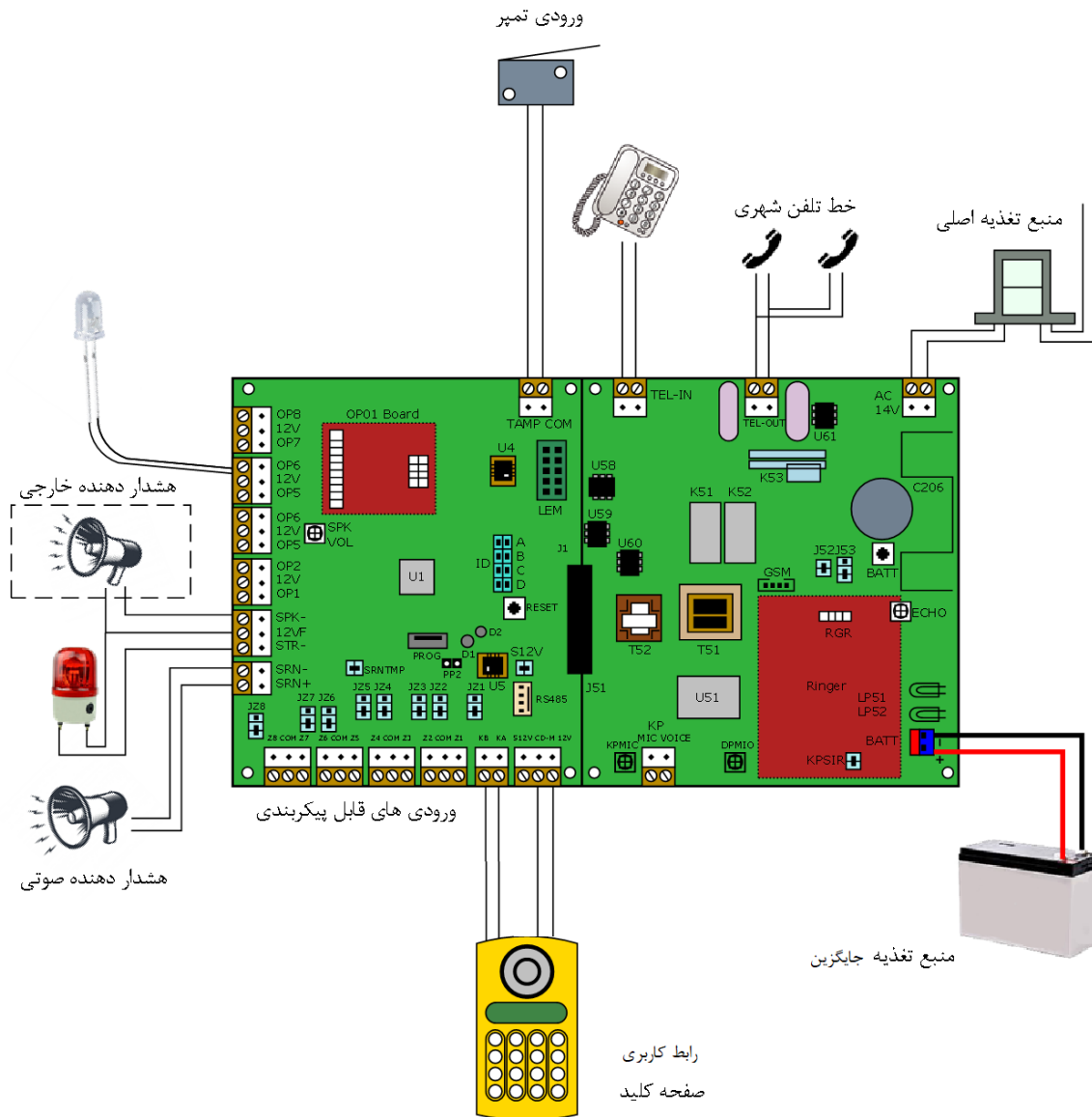
شکل ۳-۵- شمایی از یک مرکز کنترل سیستم هشدار
