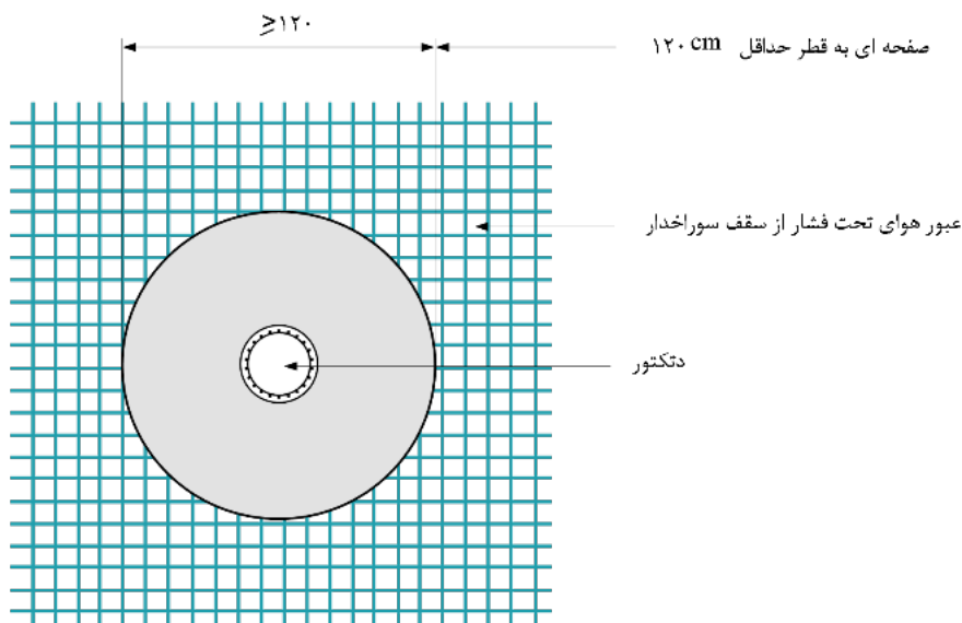
شکل ۴-۵۰- الزامات جانمایی دتکتور روی سقف‌های دارای منفذ
