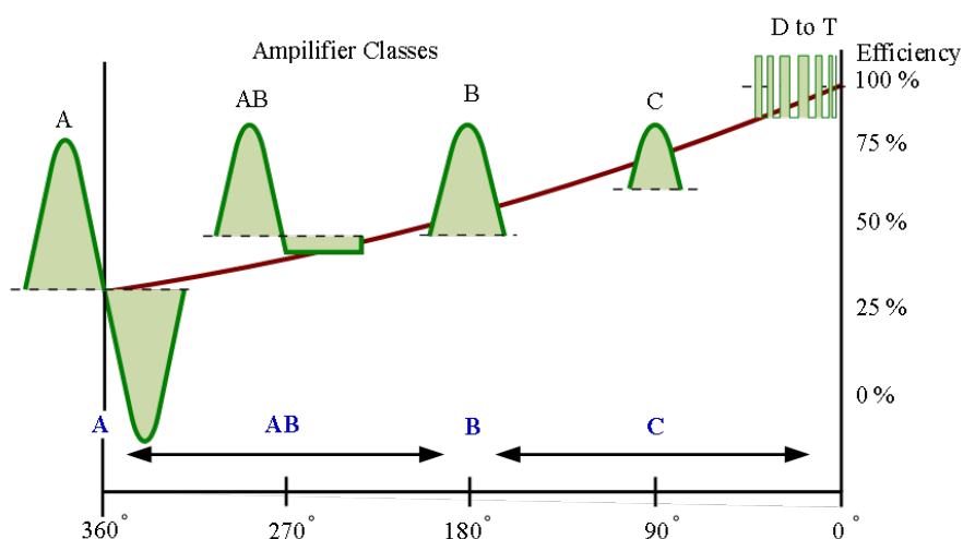
شکل ۷-۸۹- منحنی مقایسه چند کلاس مختلف از تقویت‌کننده‌ها
