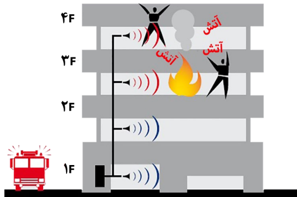
شکل ۵-۳- زون‌بندی بلندگوهای اضطراری
