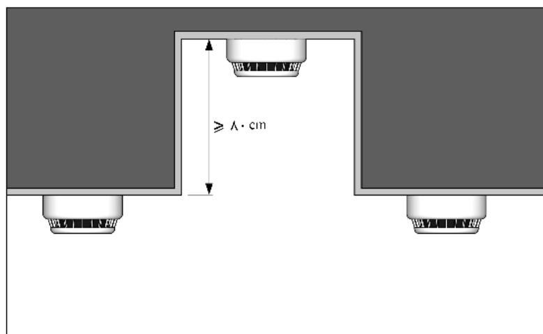
شکل ۴-۳۱- جانمایی دتکتور در نورگیر سقفی
