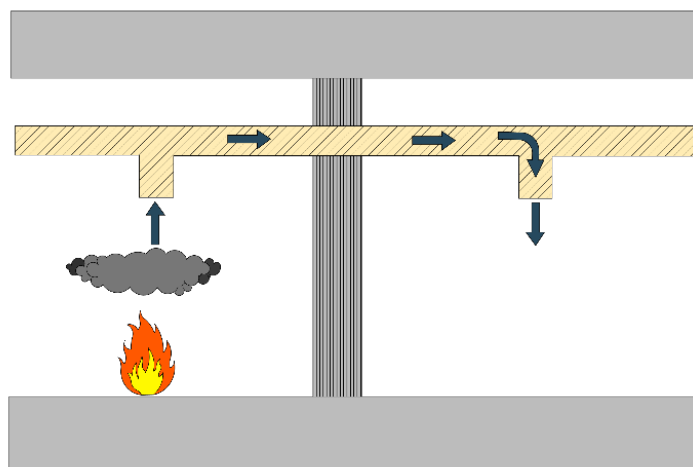
شکل ۴-۶۳- تصرفی بدون استفاده از دکتور کانالی - شروع حریق از واحد سمت چپ
