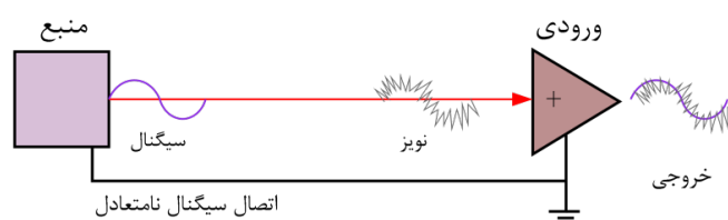
شکل ۷-۹- ارتباط منبع سیگنال با ورودی دستگاه به وسیله سیگنال نامتعادل
