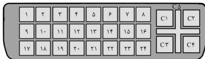
شکل ۸-۲۵- نمای روبروی سوکت مادگی DVI-I
