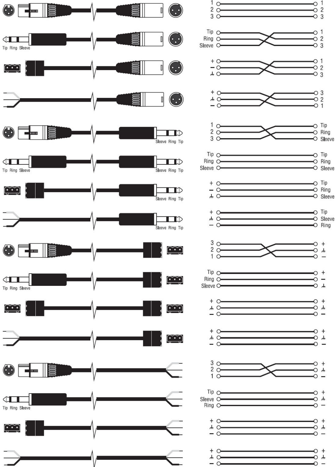
شکل ۷-۱۵۶- نحوه اتصال خروجی سیگنال متوازن به ورودی متوازن با اتصالات مختلف
