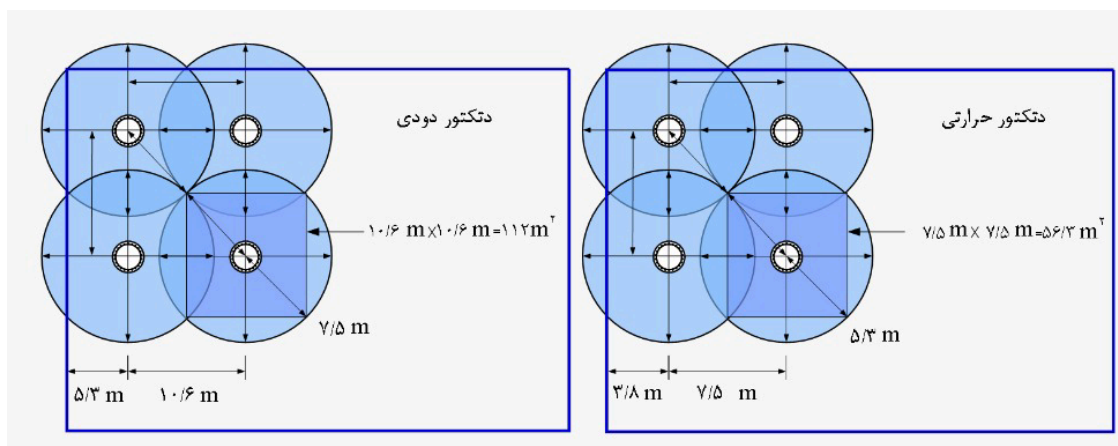
شکل ۴-۳۳- محدوده پوشش دکتورهای دودی و حرارتی نقطه‌ای
