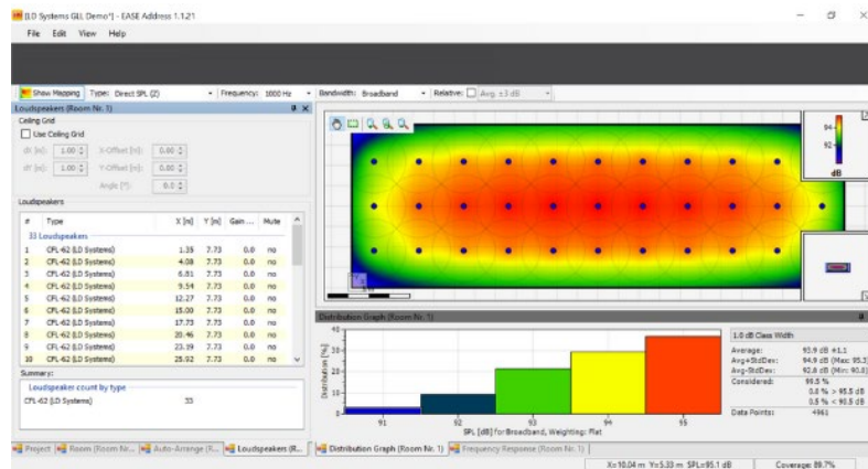
شکل ۷-۱۶۱- یک نمونه نرم‌افزار طراحی سیستم صوتی
