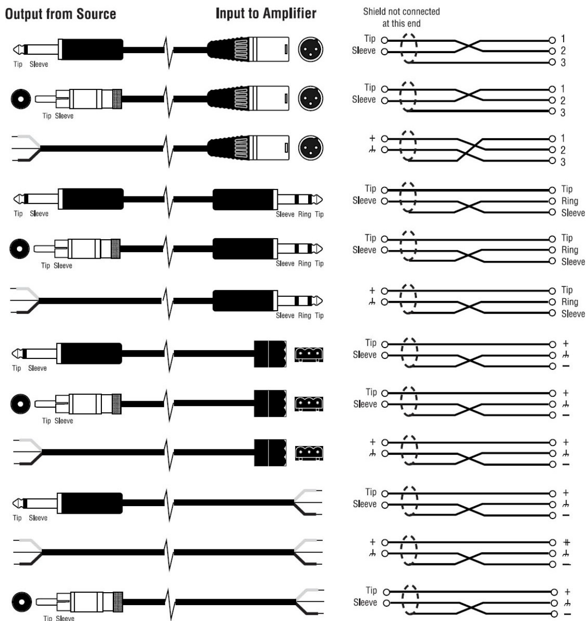
شکل ۷-۱۵۷- نحوه اتصال خروجی سیگنال نامتوازن به ورودی متوازن با اتصالات مختلف
