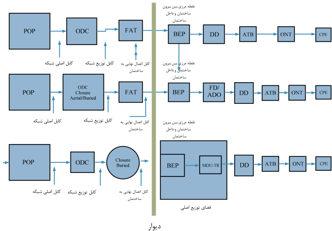
شکل ۱۶-۱- نمونه‌هایی از اصطلاحات طراحی شبکه فیبر نوری ساختمان‌ها در ایران
