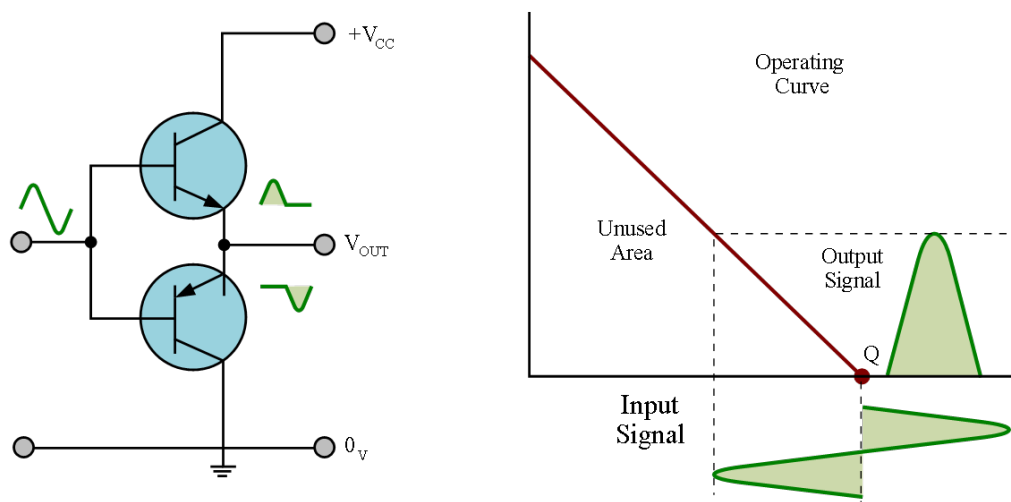
شکل ۷-۹۱- یک نمونه مدار ساده و منحنی نقطه کار و خط بار تقویت کننده کلاس B
