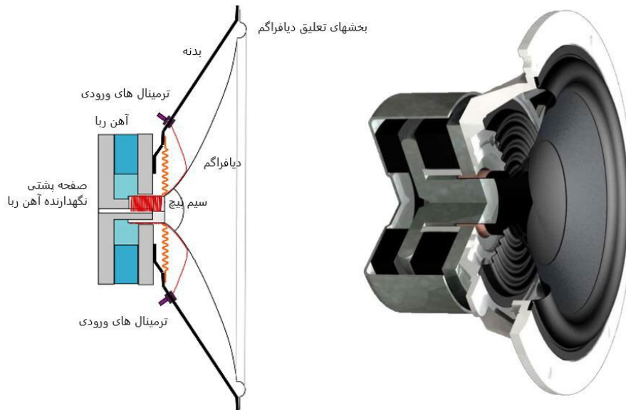
شکل ۷-۱۰۹- ساختمان داخلی یک بلندگو با واحد راه‌انداز داینامیک
