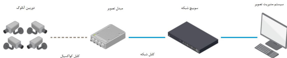
شکل ۳-۲۹- یک نمونه استفاده از مبدل جهت تبدیل ویدیوی آنالوگ دریافتی به ویدیوی دیجیتال
