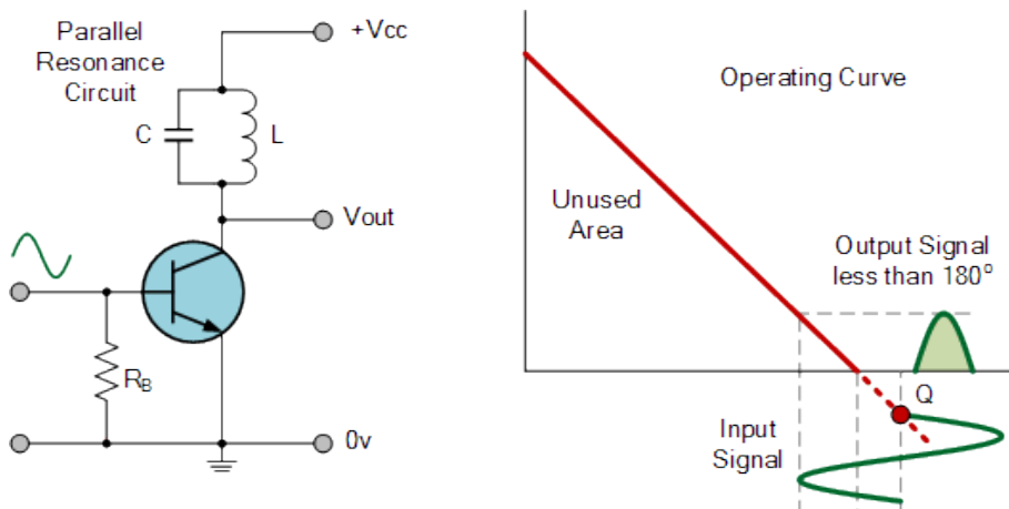
شکل ۷-۹۳- یک نمونه مدار ساده و منحنی نقطه کار و خط بار تقویت‌کننده کلاس C
