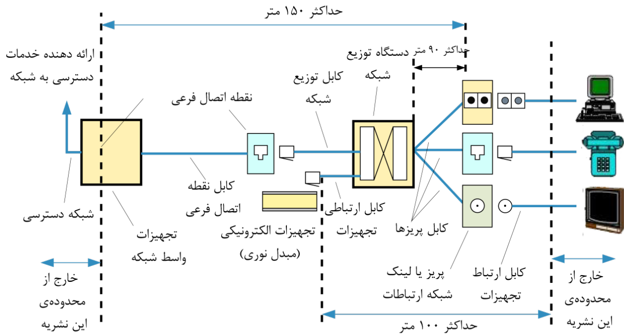
شکل ۱-۱۷- اجزای کابل کشی در یک واحد آپارتمان دوبلکس
