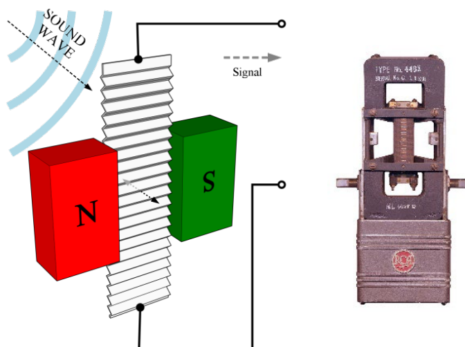
شکل ۷-۳۰- ساختمان داخلی و یک نمونه کپسول میکروفن نواری
