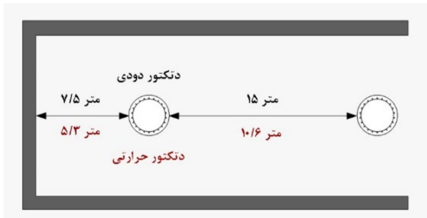
شکل ۴-۳۴- جانمایی دکتور دودی در راهروهای با عرض کم‌تر از ۲ متر
