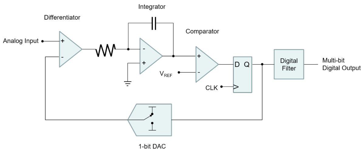
شکل ۷-۱۴- بلوک دیاگرام مبدل آنالوگ به دیجیتال سیگما دلتا
