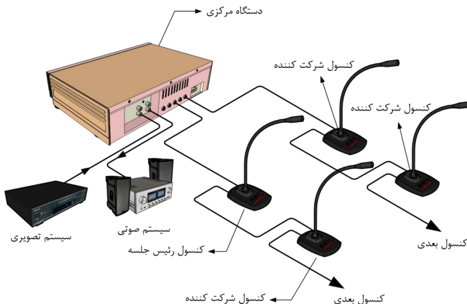
شکل ۸-۲- اجزاء یک سیستم کنفرانسی ساده
